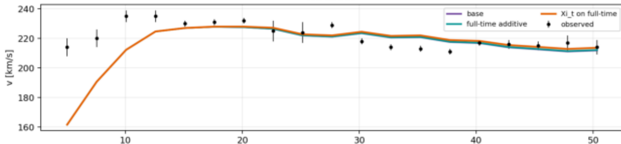
NGC7331
