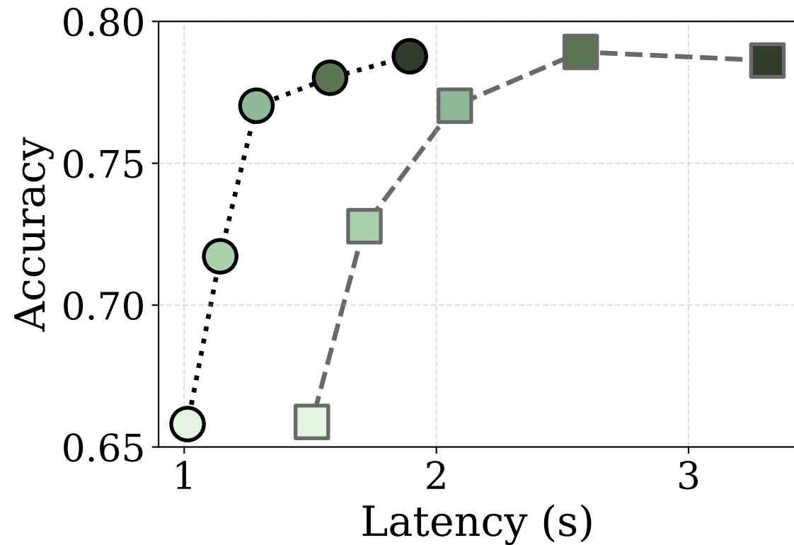
GSM8K
