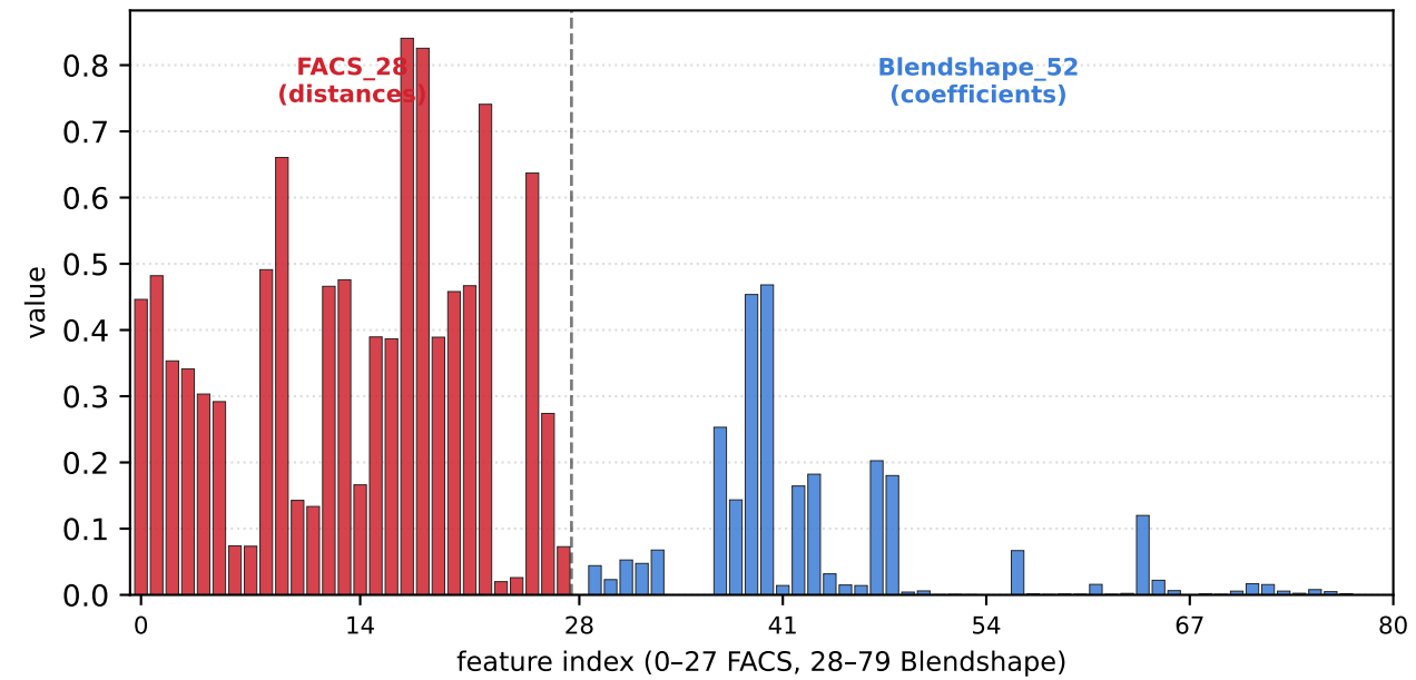
(d) facs_plus_bs_80 — concat 28 jarak FACS + 52 koefisien Blendshape
