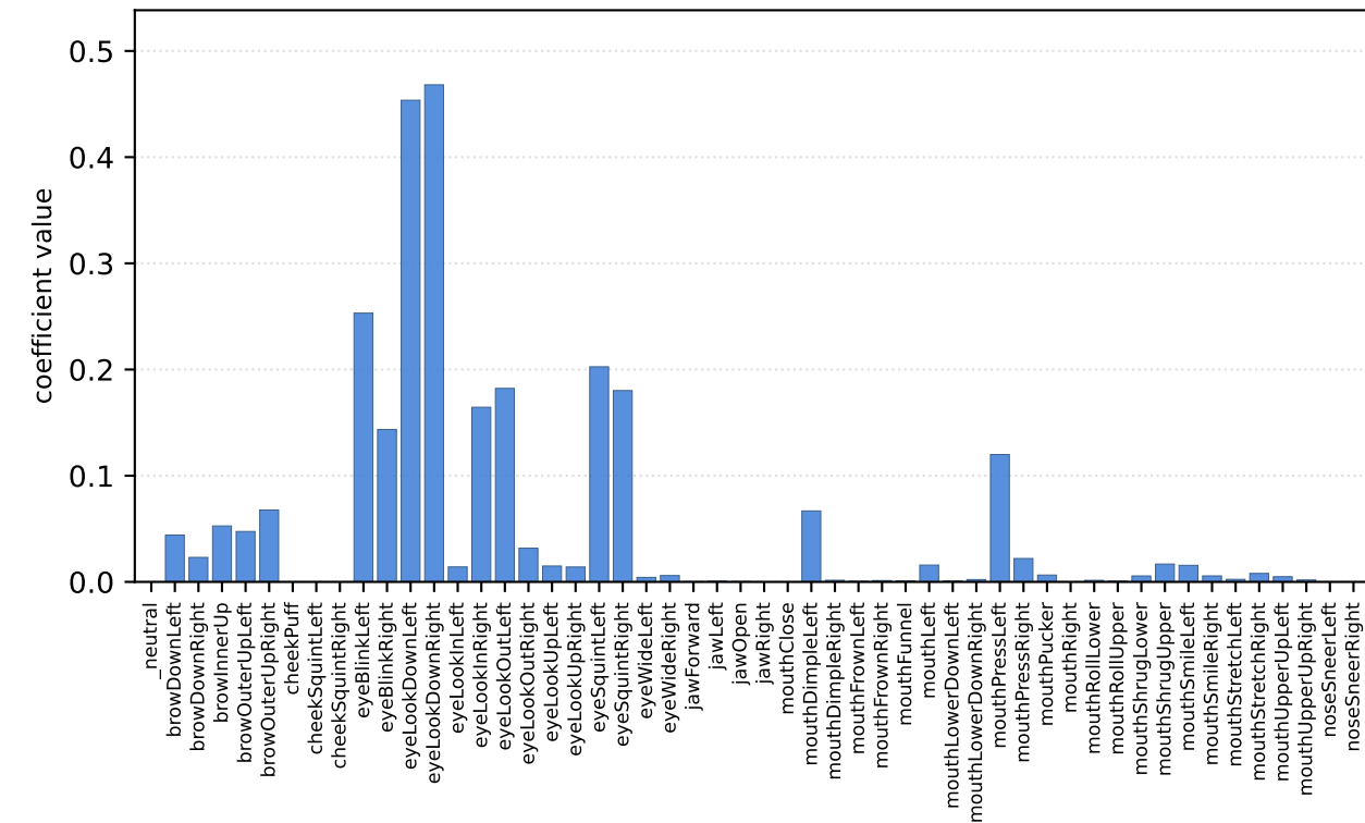
(c) blendshape_52 — 52 koefisien ARKit (MediaPipe FaceLandmarker v2)
