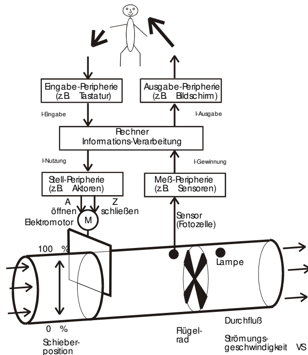
Bild 1_30: Objekte und Systeme in der Gebäudeautomation
