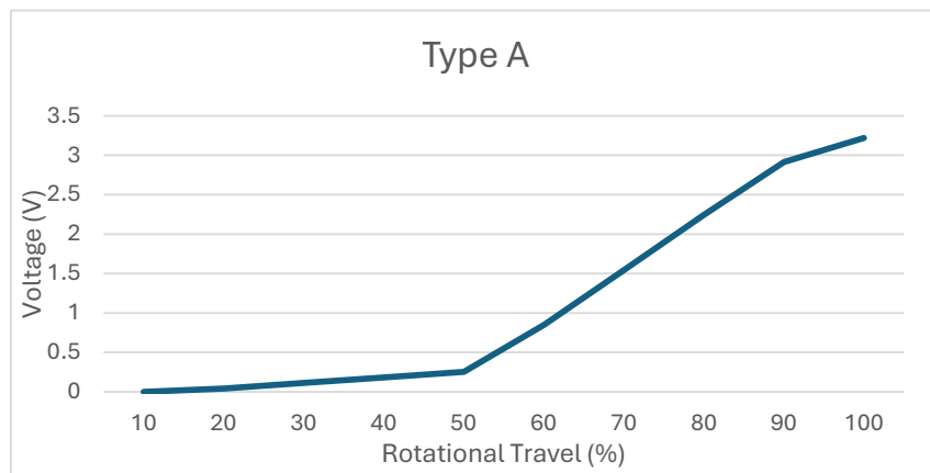
รูปที่ 3 กราฟแสดงความสัมพันธ์ของแรงดันขาออกกับตำแหน่งตัวหมุนของ Type A
