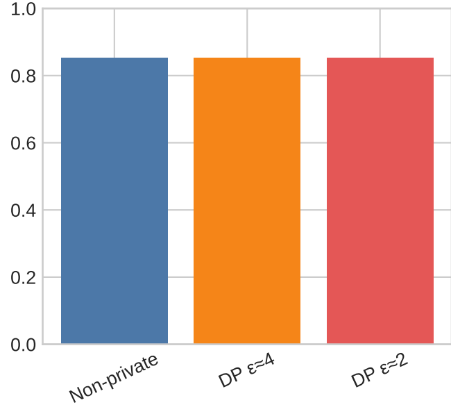
F1
