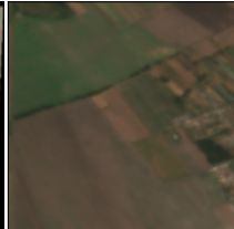
Planet (3 m)
