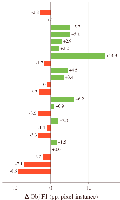
FTW pixel-instance Obj F1
