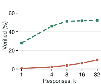
Llama 3.1-8B
