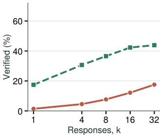
Qwen3-30B-A3B
