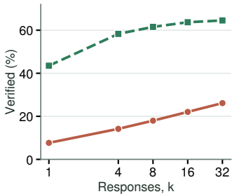
Qwen3-14B
