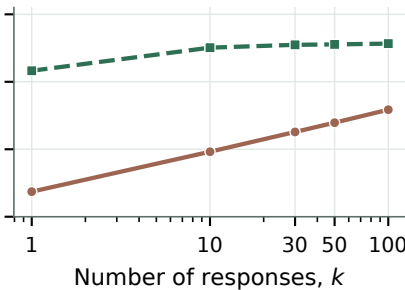
(e) Qwen3-30B-A3B
