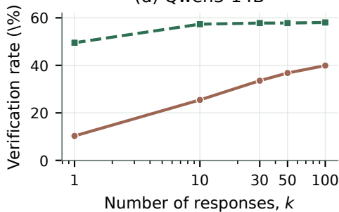
(d) Qwen3-14B
