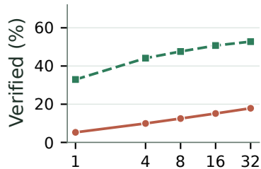
(a) Qwen3-4B
