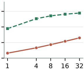
(b) Qwen3-8B
