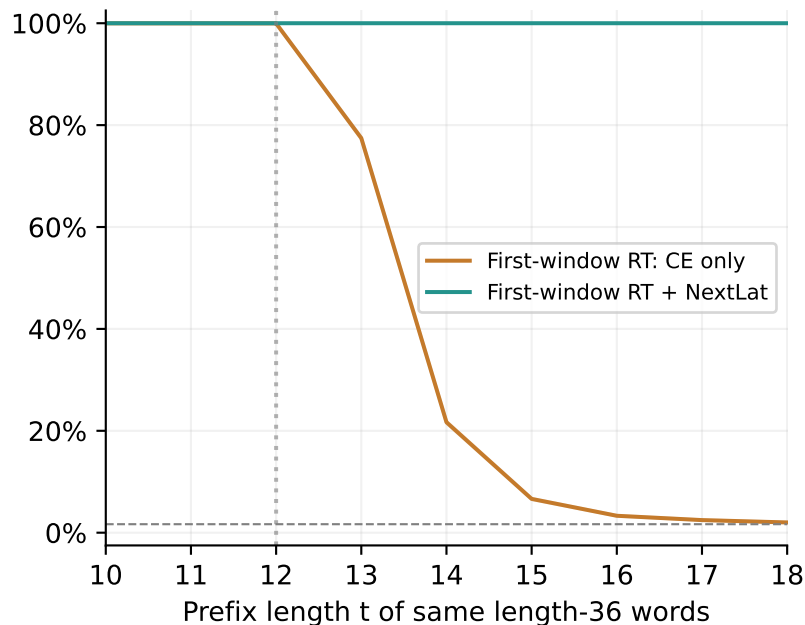
A: state t correct
