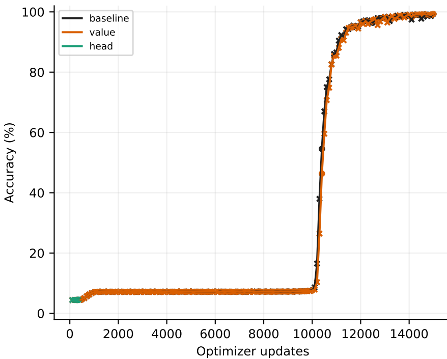
A5 L36: Token
