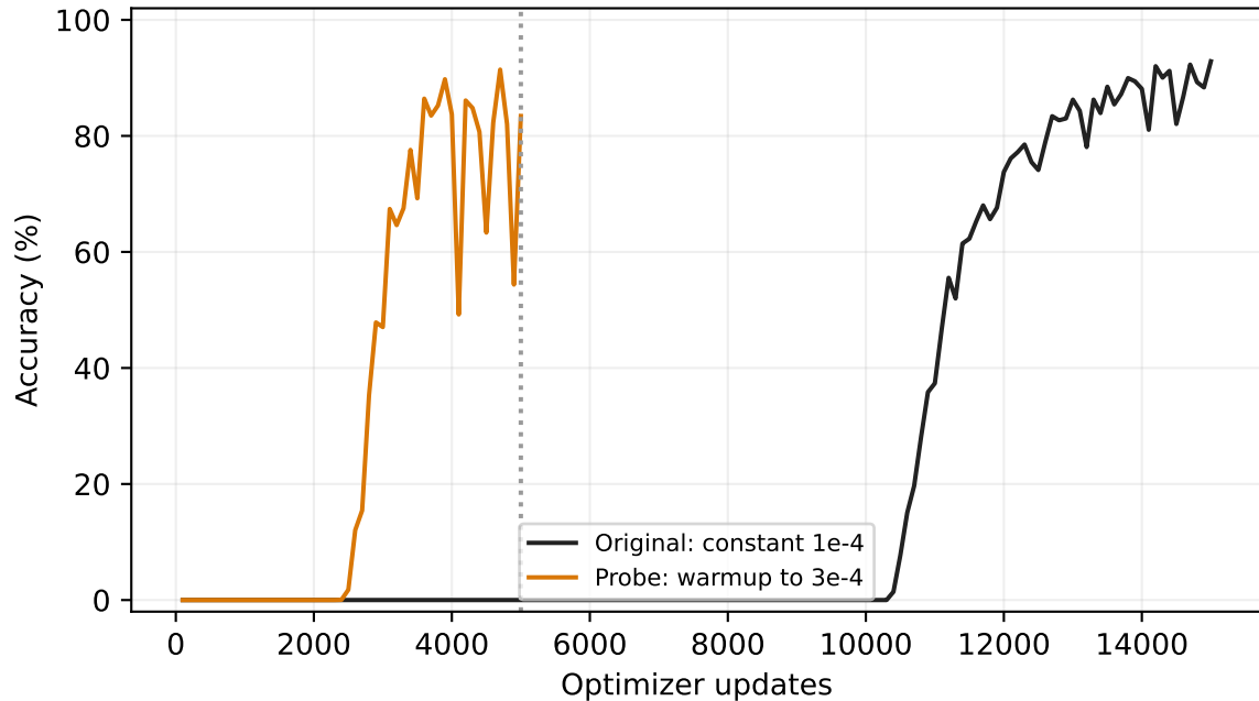
A5 length36 whole word
