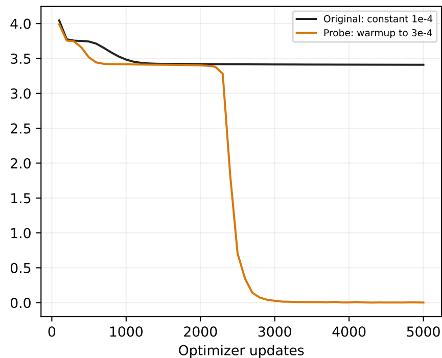
A5 NextLat loss
