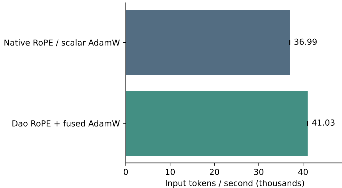
B16 / T2048
