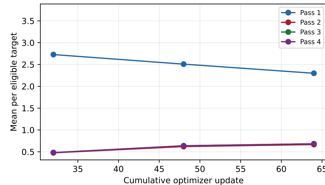
NFR KL1: raw KL
