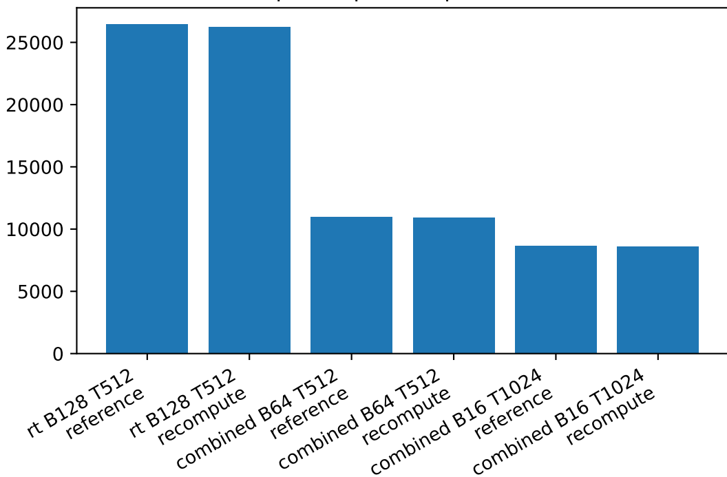
Complete-update input tokens/s
