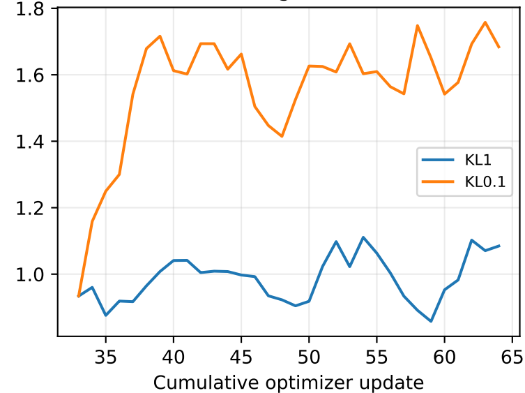
Training raw KL
