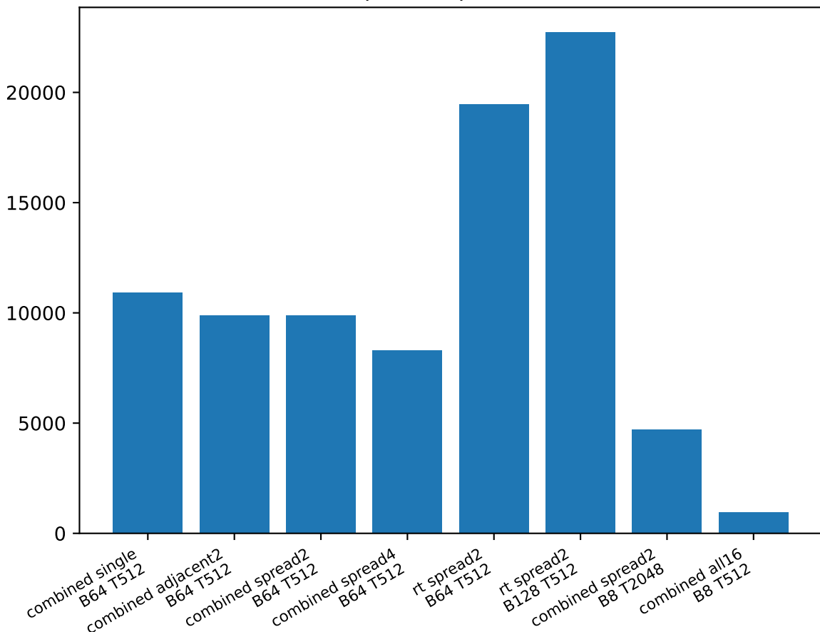
Full-update input tokens/s
