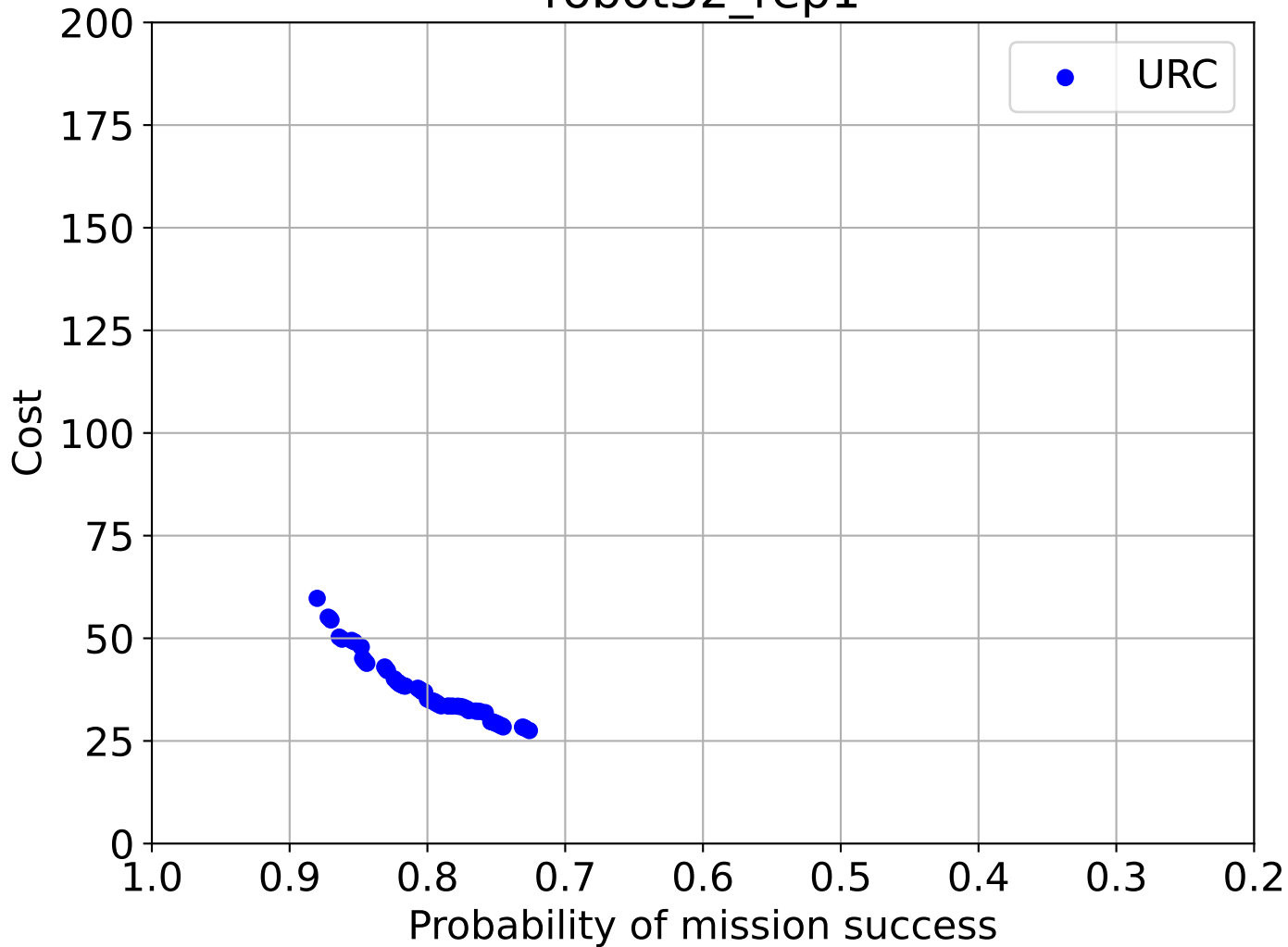
robot32_rep1
