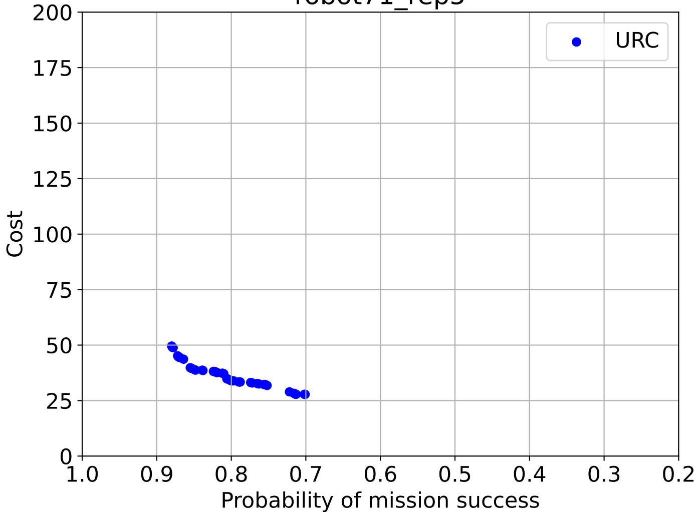
robot71_rep5
