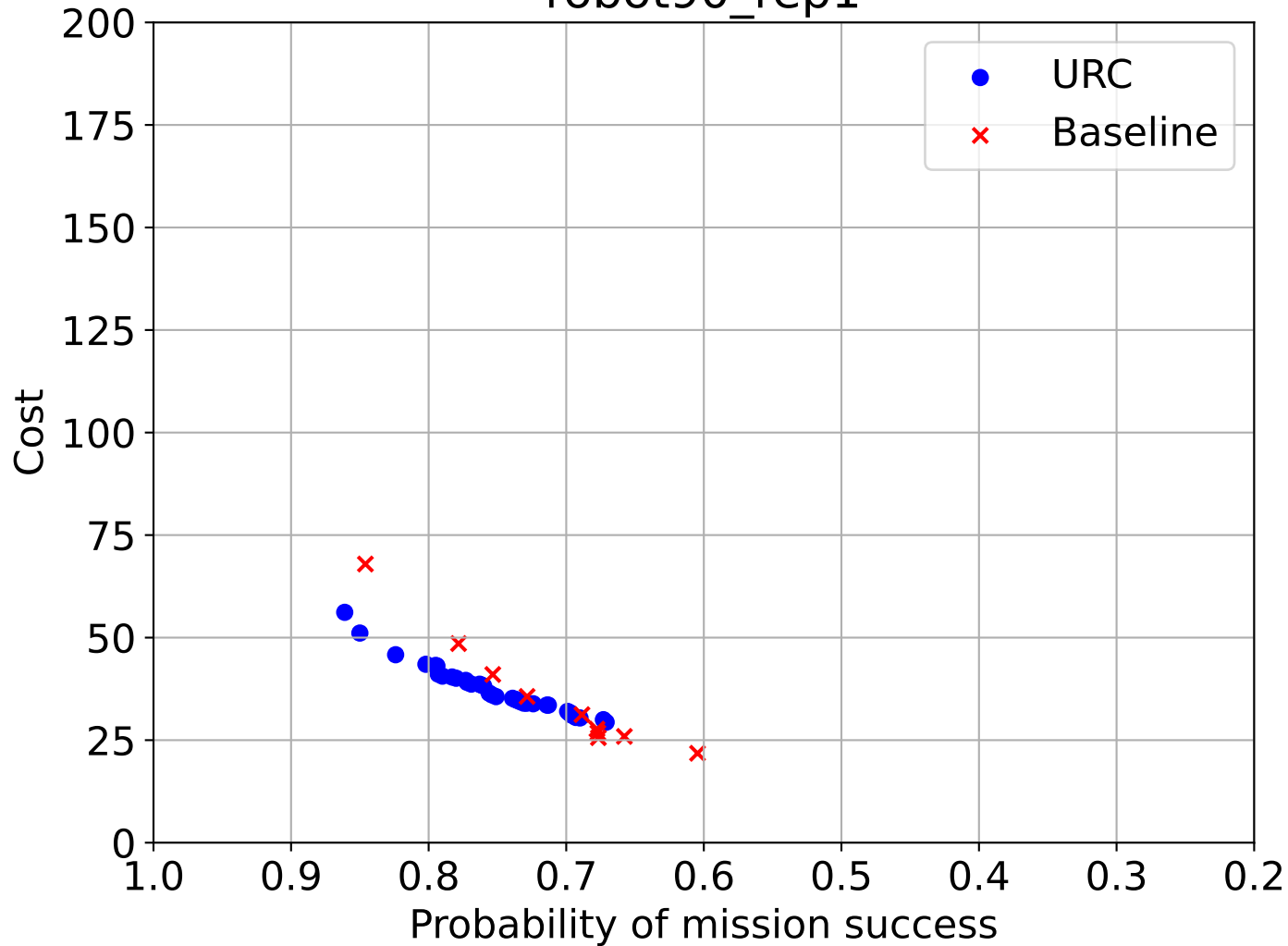
robot90_rep1
