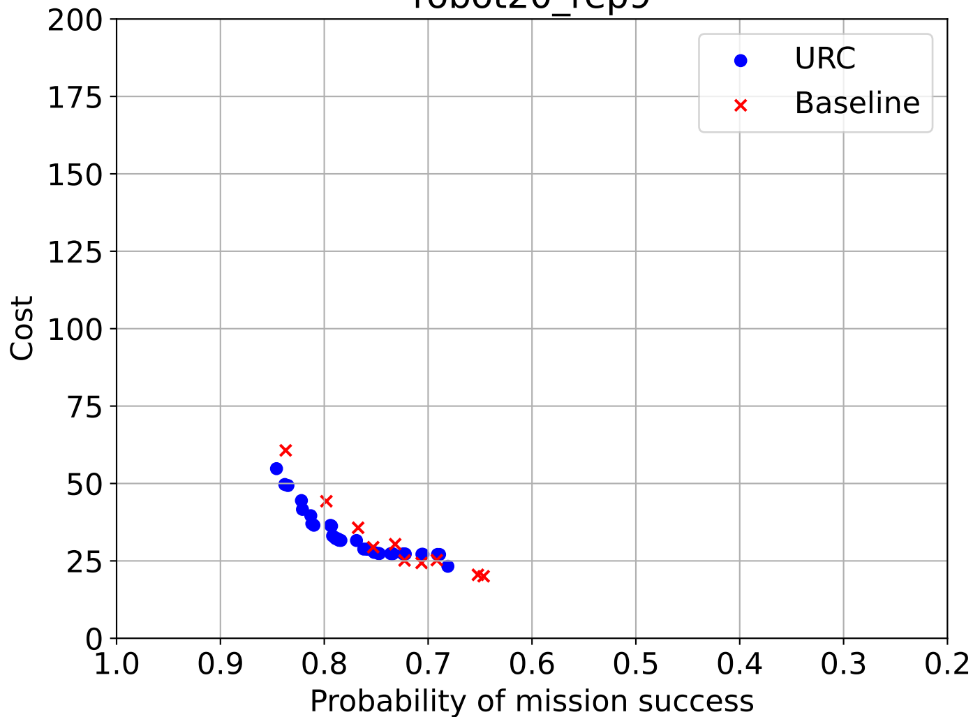
robot20_rep9
