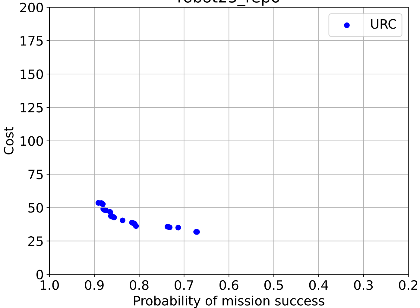
robot23_rep6
