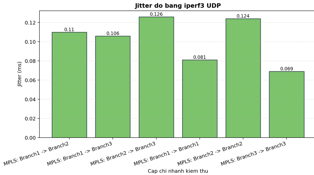
Hình 4.5 Jitter đo bằng iperf3 UDP
