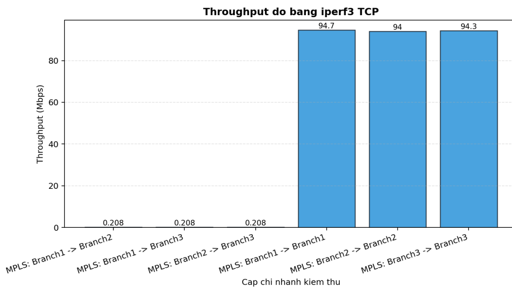
Hình 4.2 Throughput đo bằng iperf3 TCP
