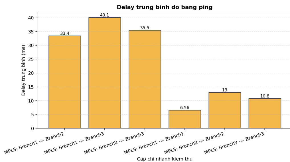
Hình 4.3 Delay trung bình đo bằng ping
