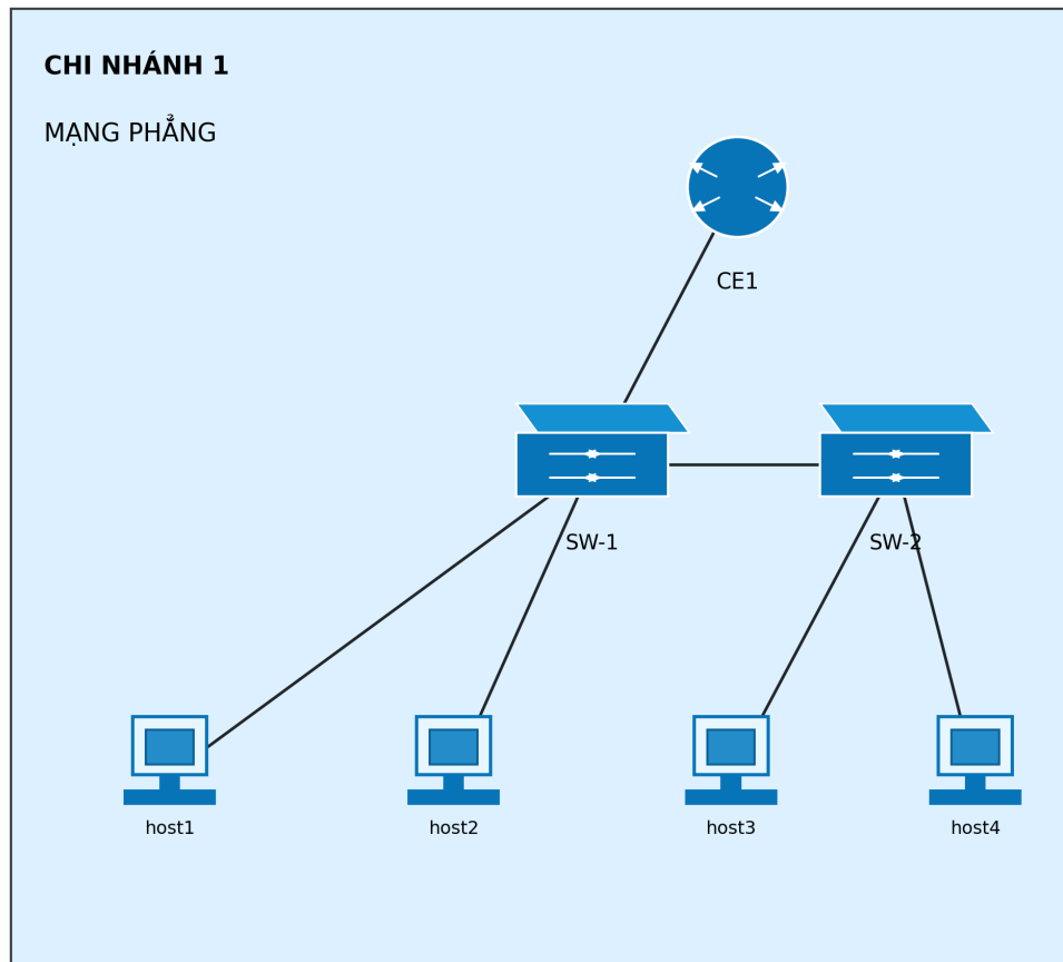
Hình 3.2 Branch 1 Flat Network
