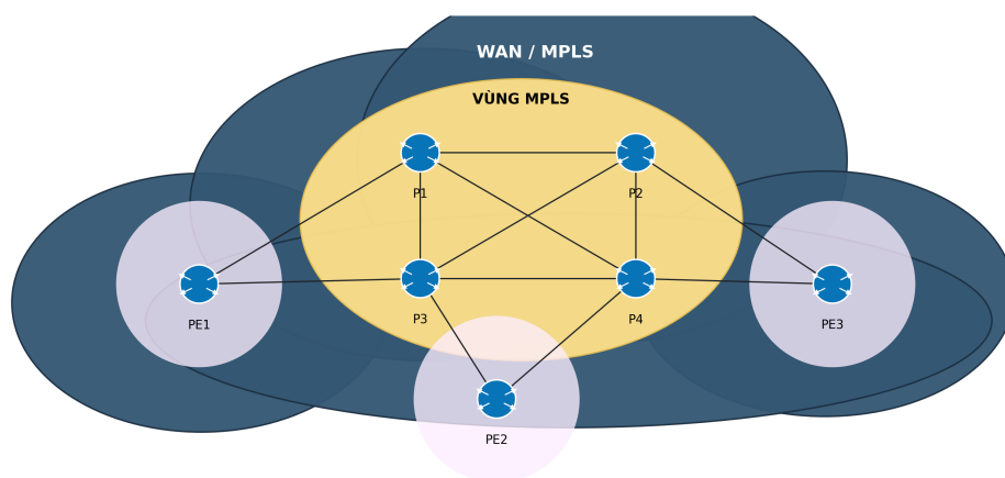
Hình 3.5 Provider MPLS backbone
