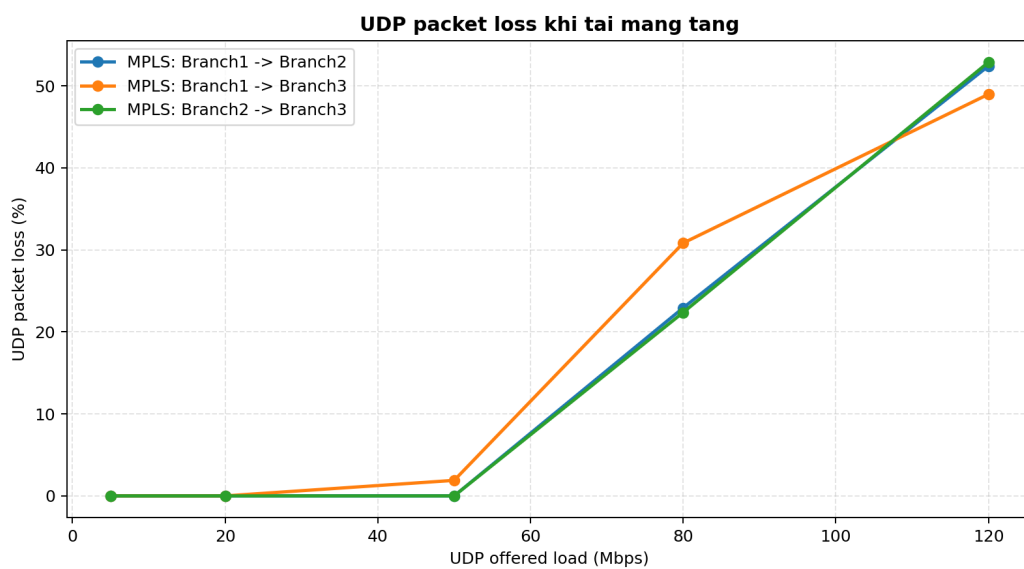
Hình 4.4 UDP packet loss khi tải mạng tăng
