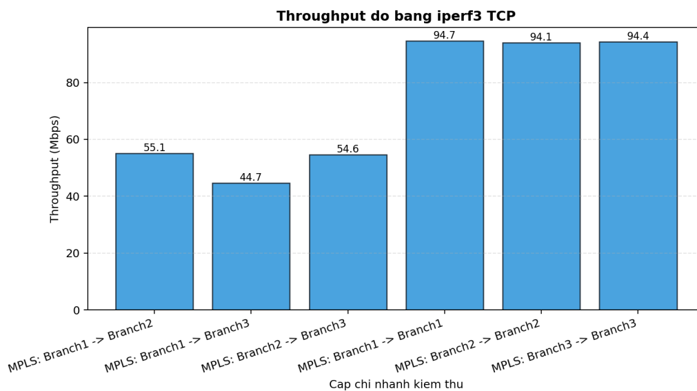
Hình 4.1 Throughput đo bằng iperf3 TCP
