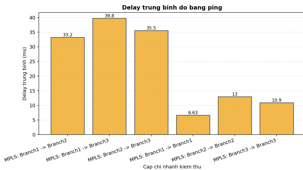
Hình 4.2 Delay trung bình đo bằng ping
