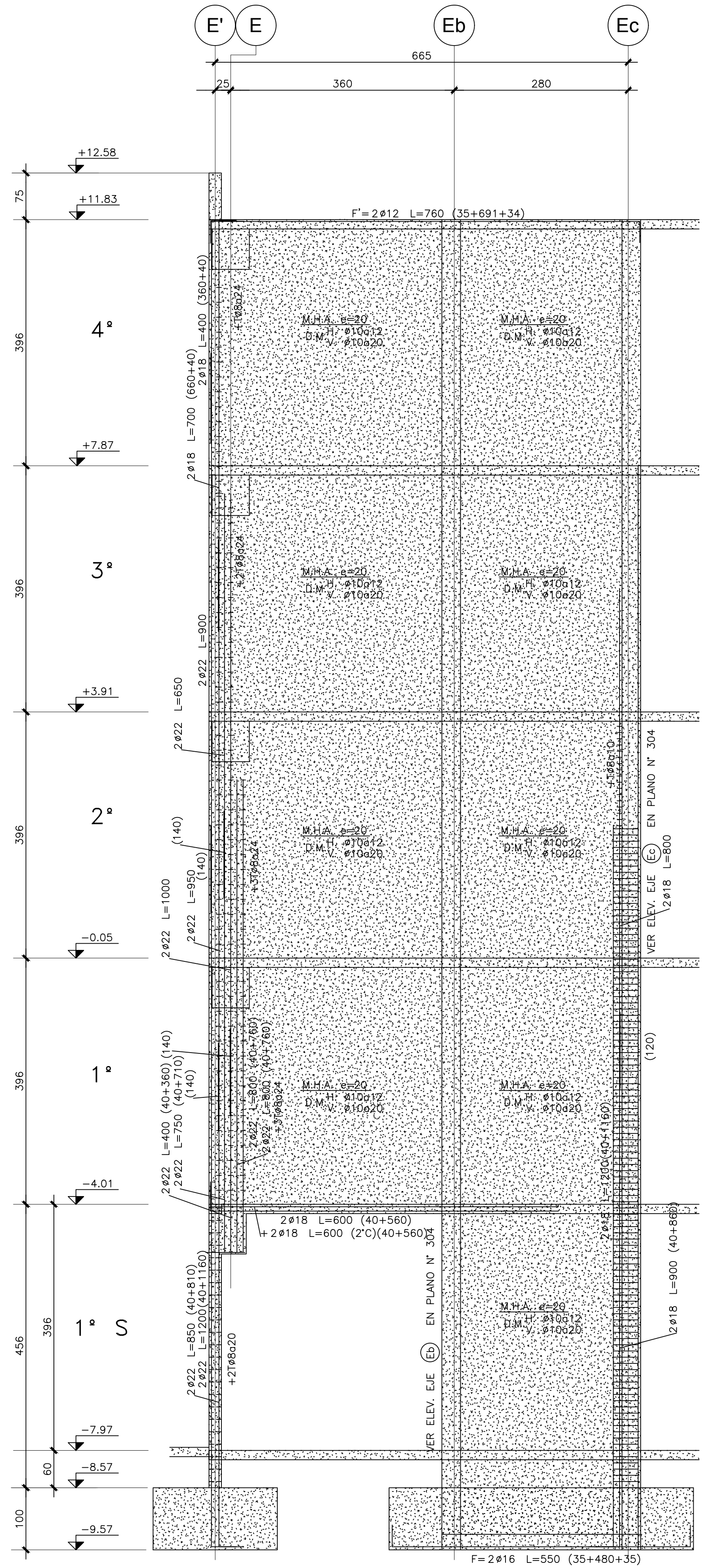
ELEVACION EJE 1''
