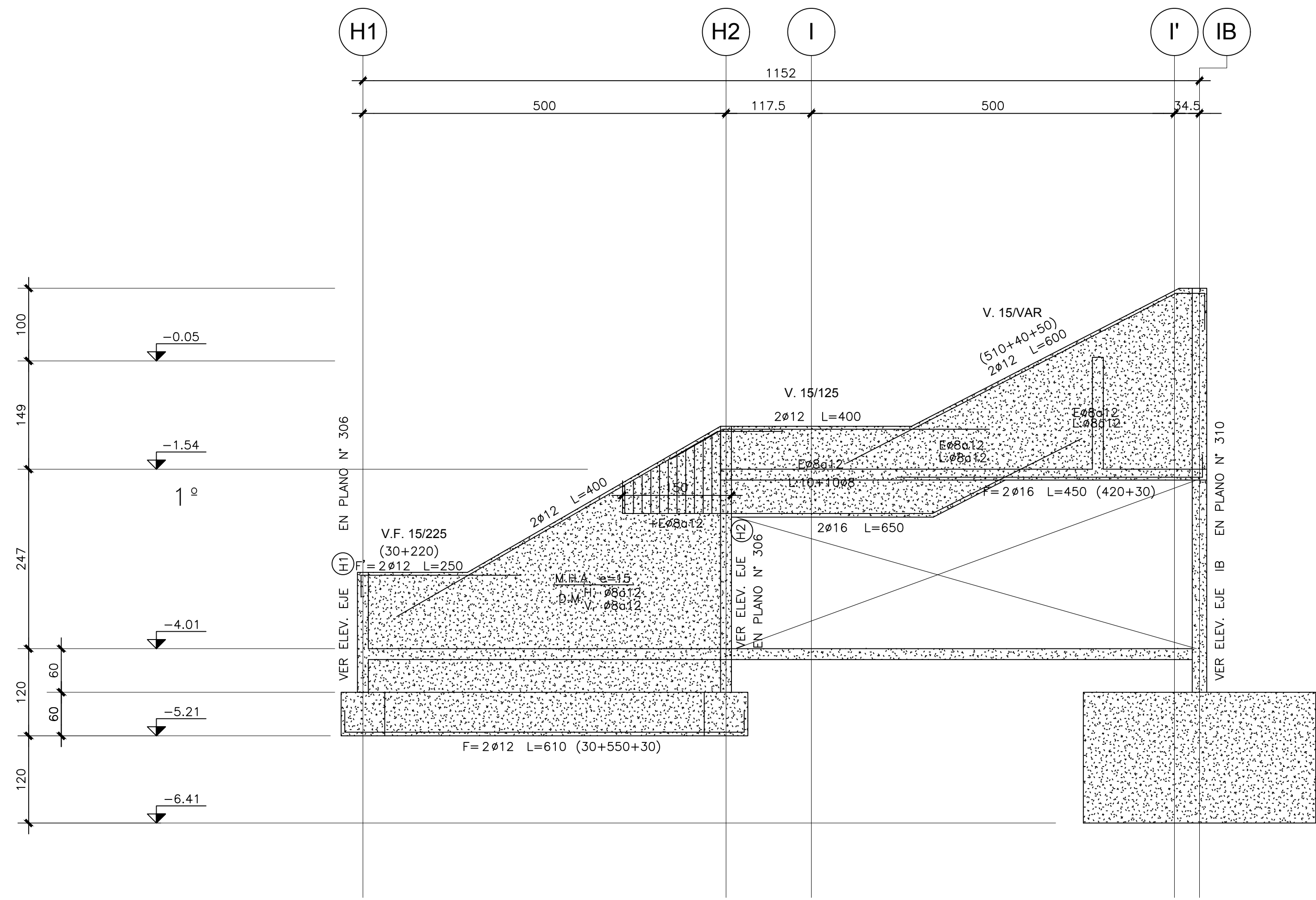
ELEVACION EJE 1A
