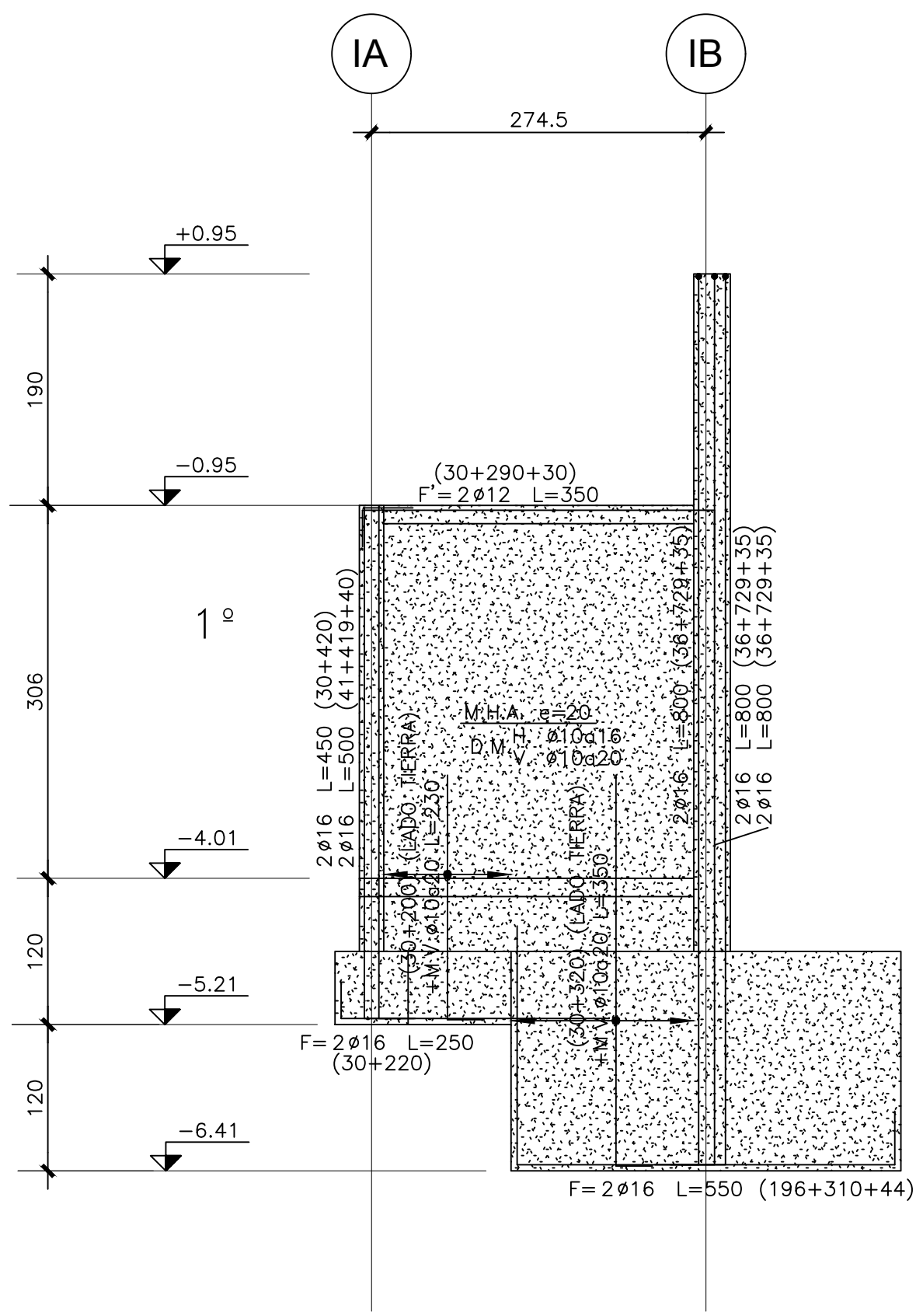
ELEVACION EJE 1C
