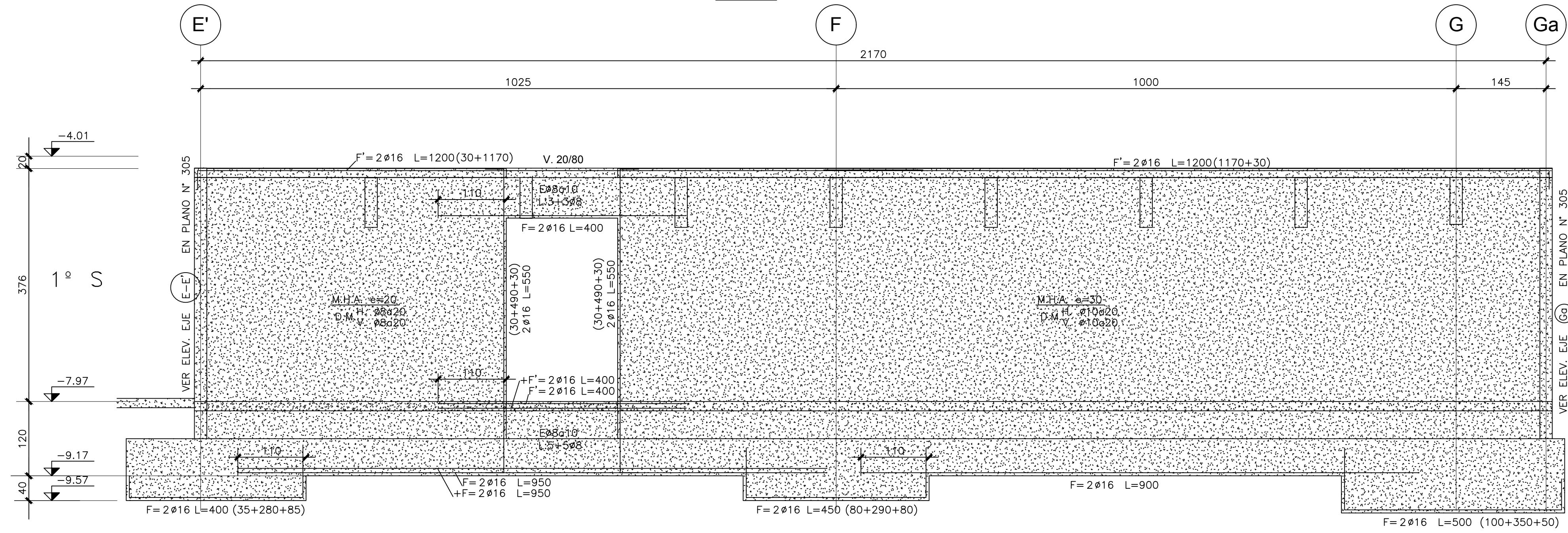
ELEVACION EJE 1A
