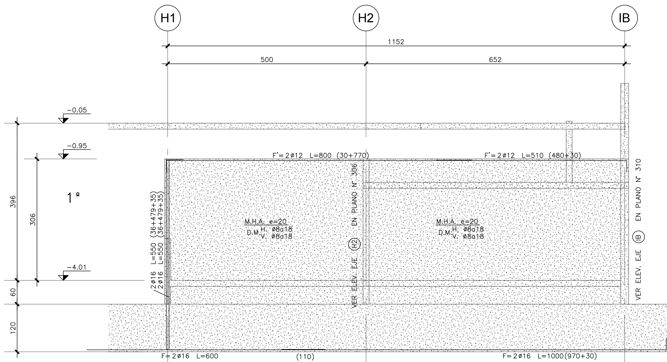
ELEVACION EJE 1AA
