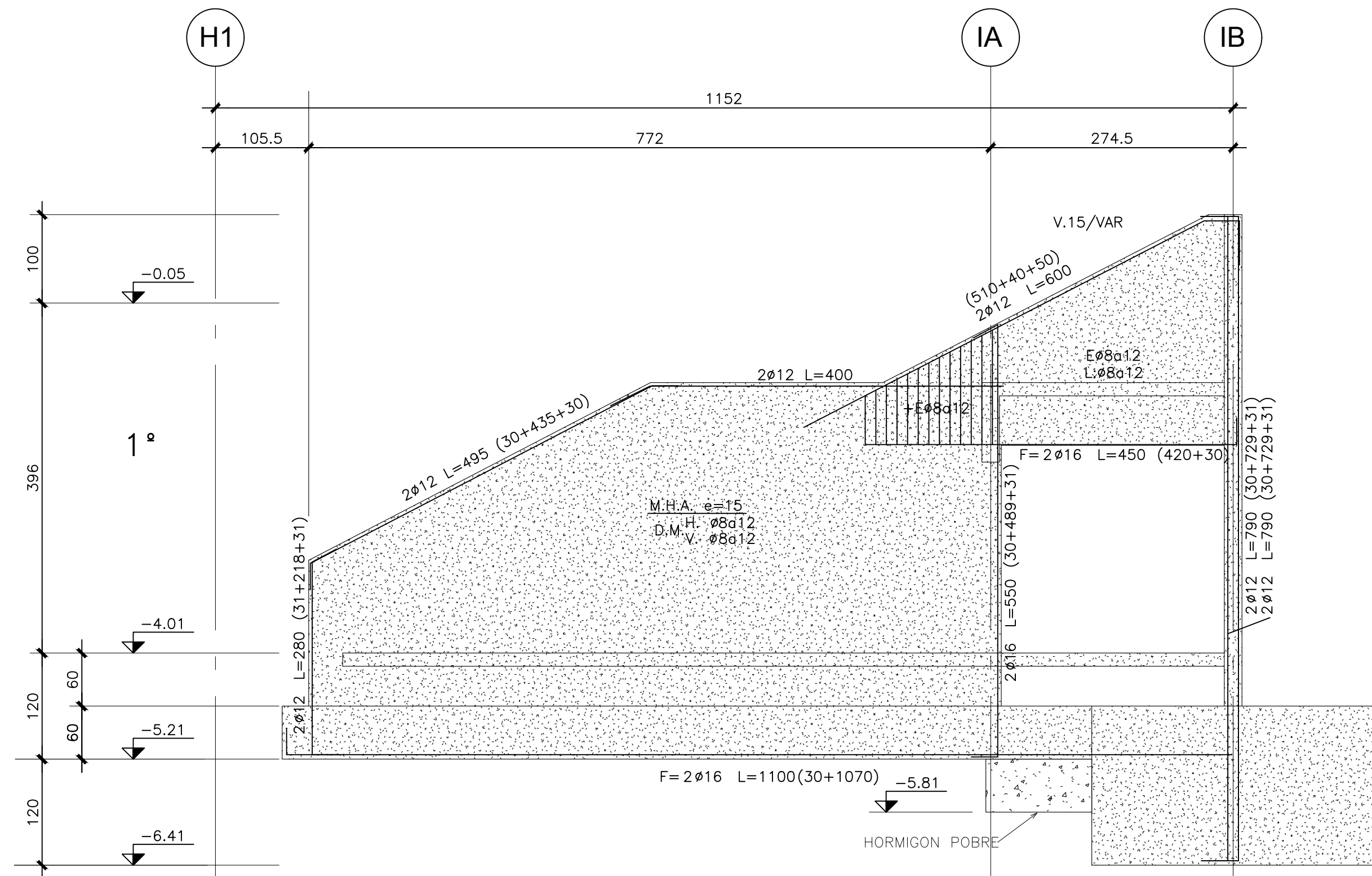
ELEVACION EJE 1BB
