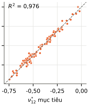
(b) Tinh chỉnh trên mật độ liên tục
