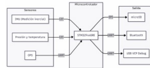
Figura 1. Diagrama en bloques del sistema.
