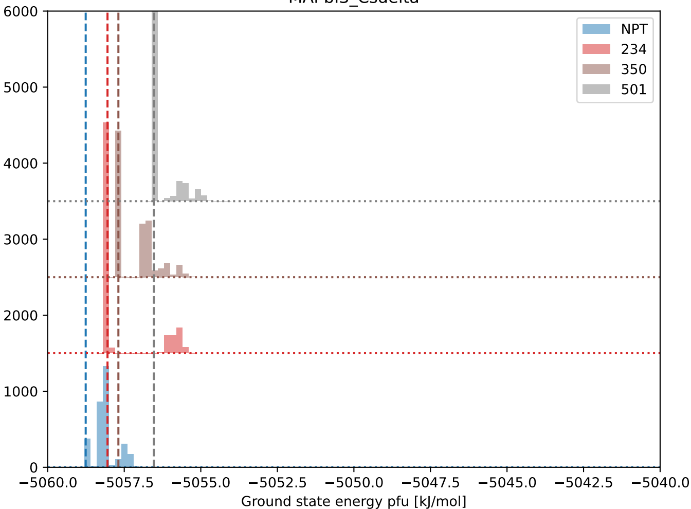
MAPbI3_Csdelta
