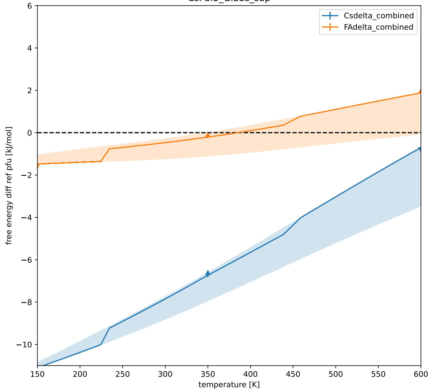
CsPbI3_Gibbs_sup
