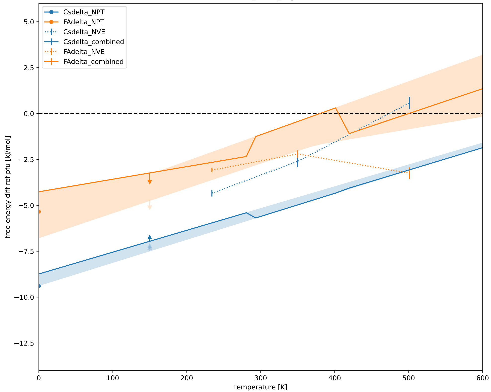
FAPbI3_Harm_sup
