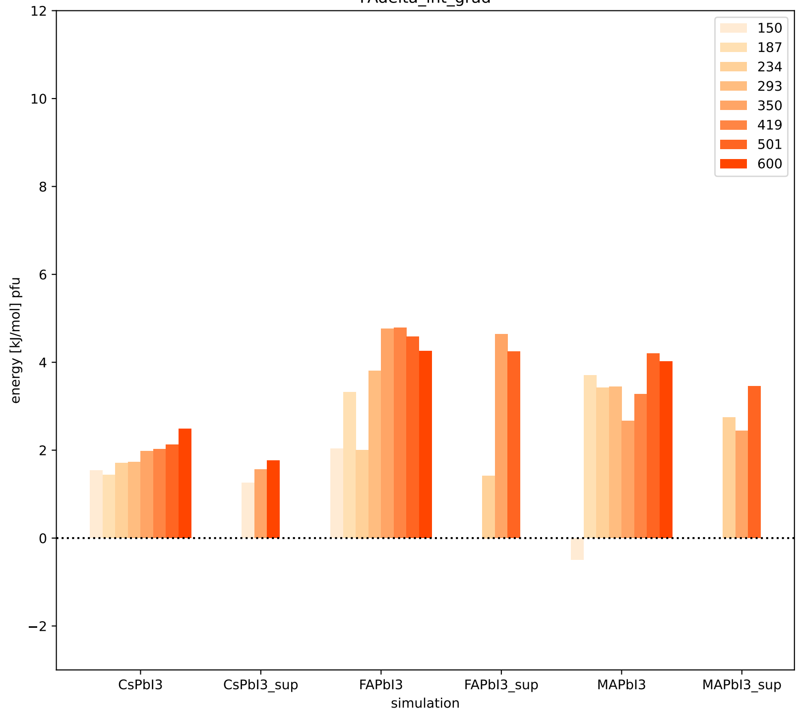
FAdelta_int_grad
