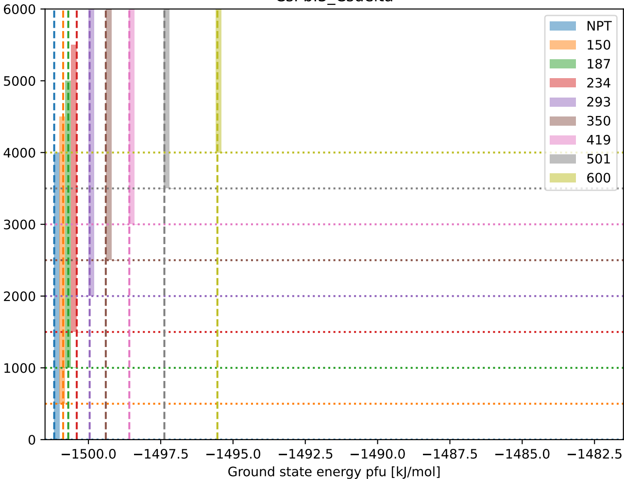
CsPbI3_Csdelta
