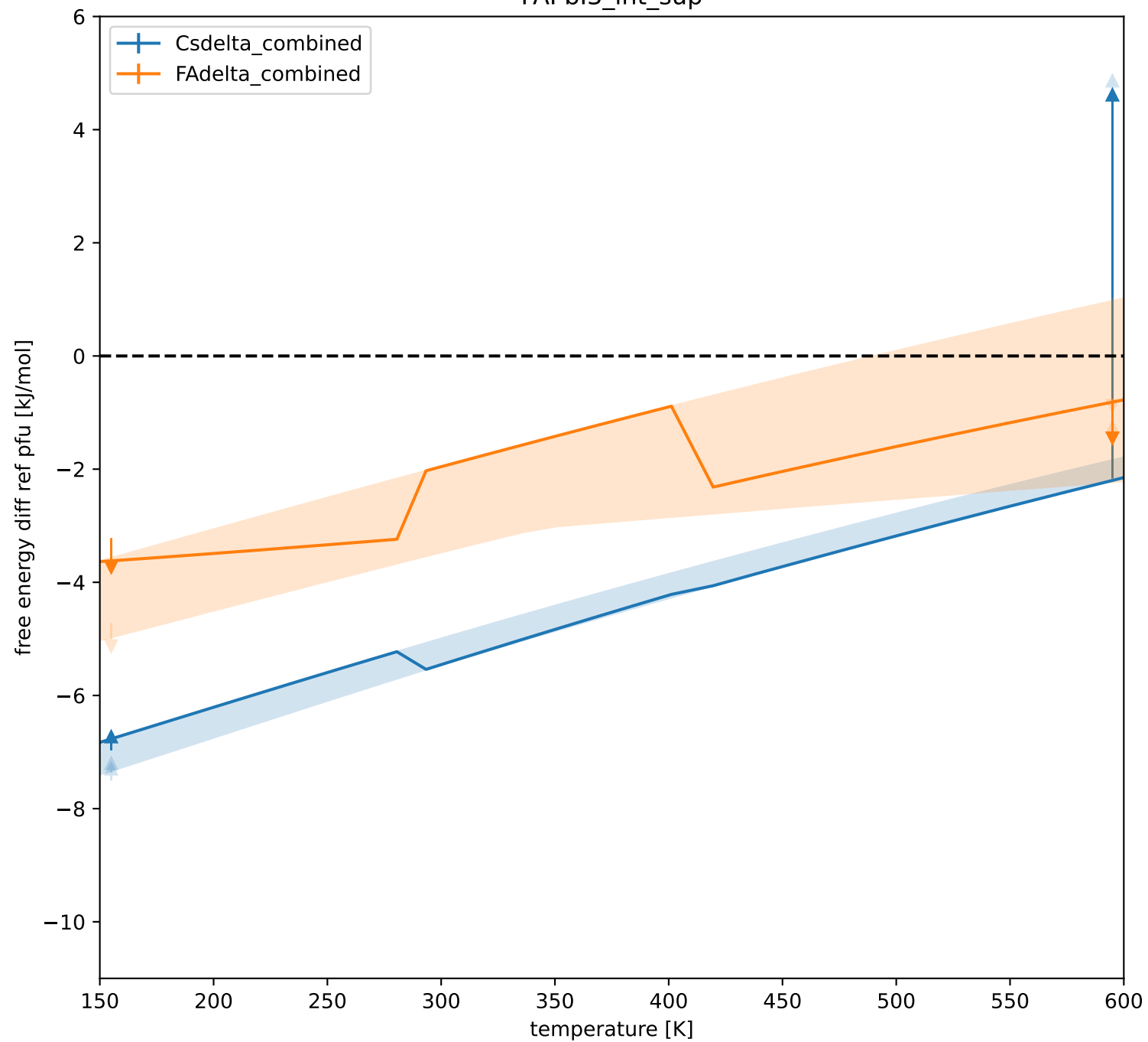
FAPbI3_int_sup
