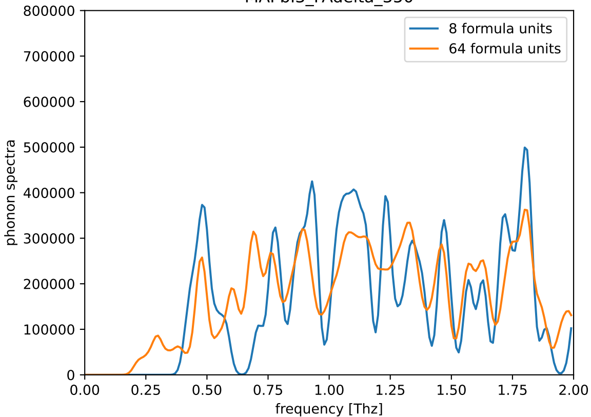
MAPbI3_FAdelta_350
