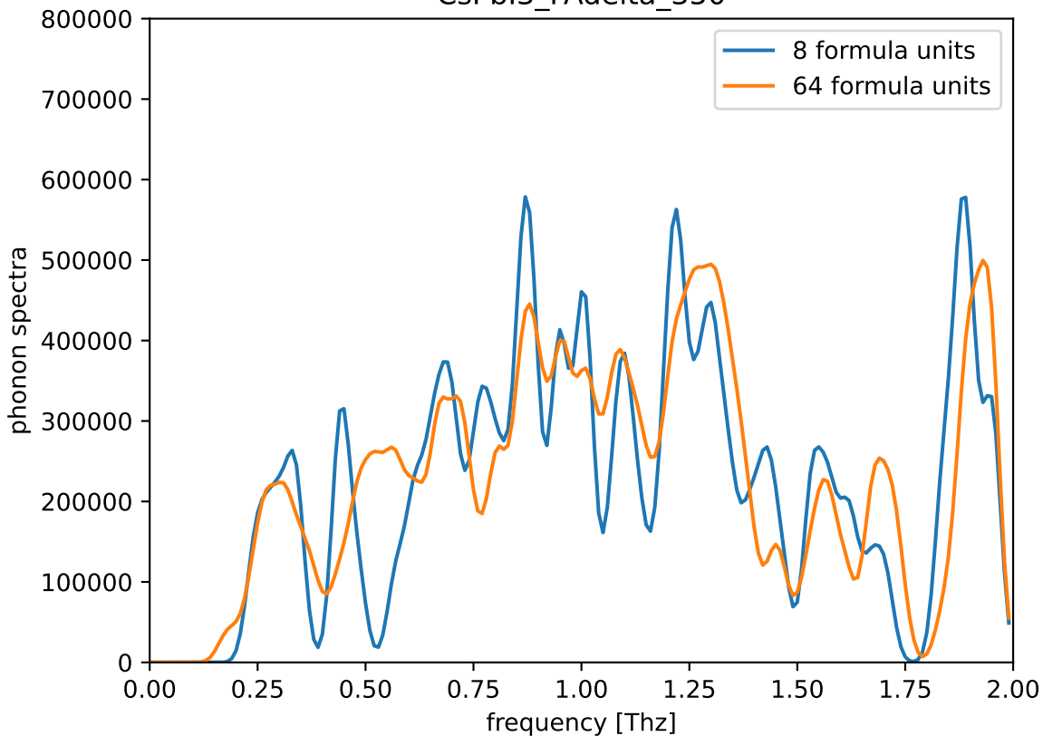
CsPbI 3 _FAdelta_350
