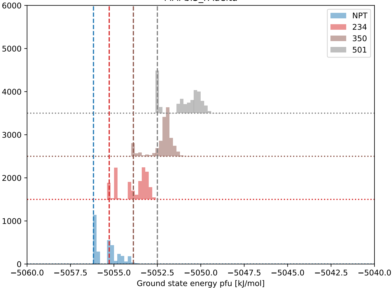
MAPbI3_FAdelta
