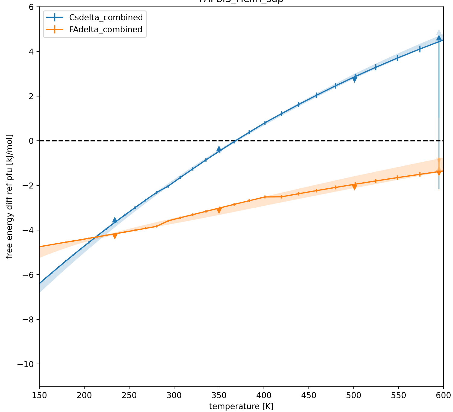
FAPbI3_Helm_sup
