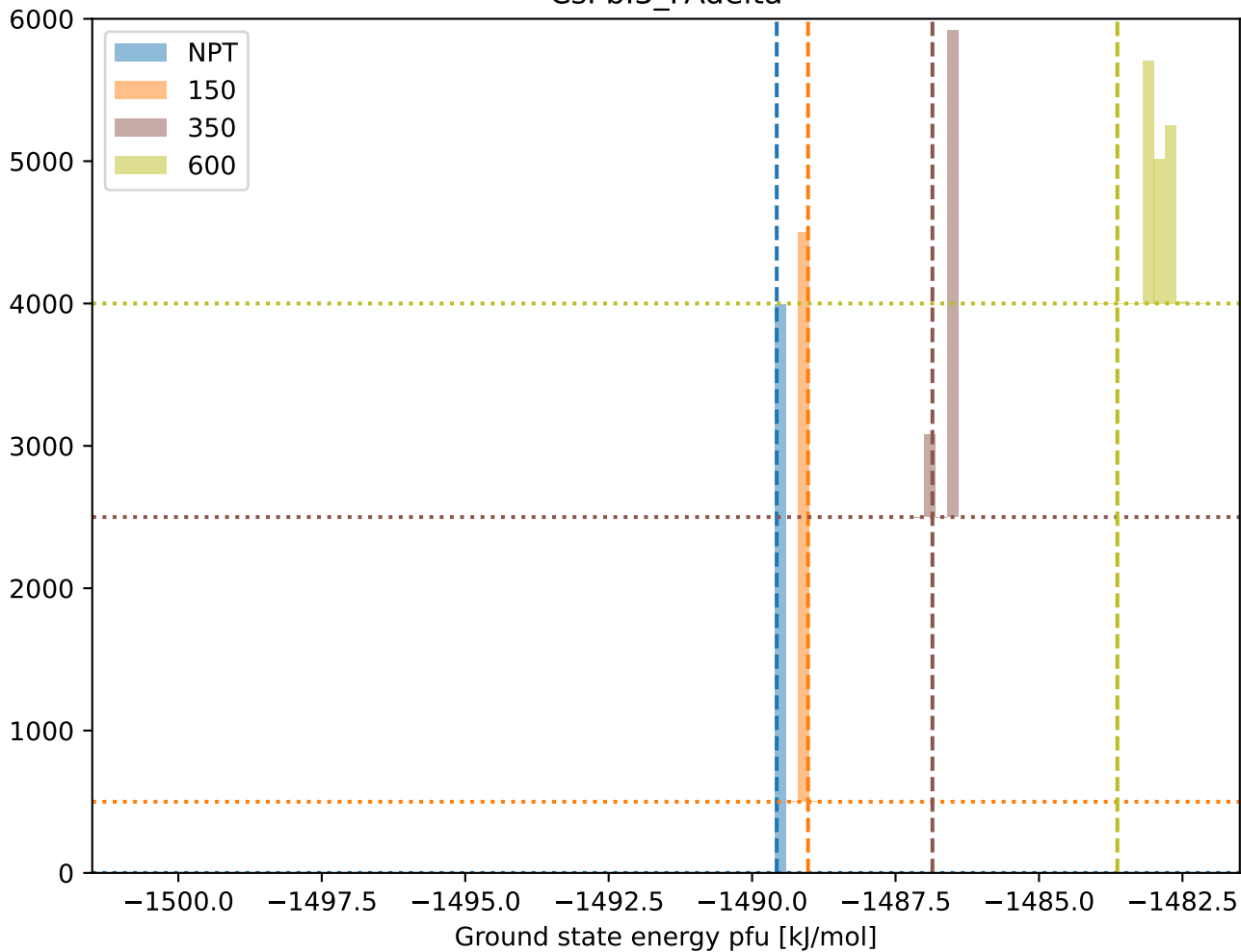
CsPbI3_FAdelta
