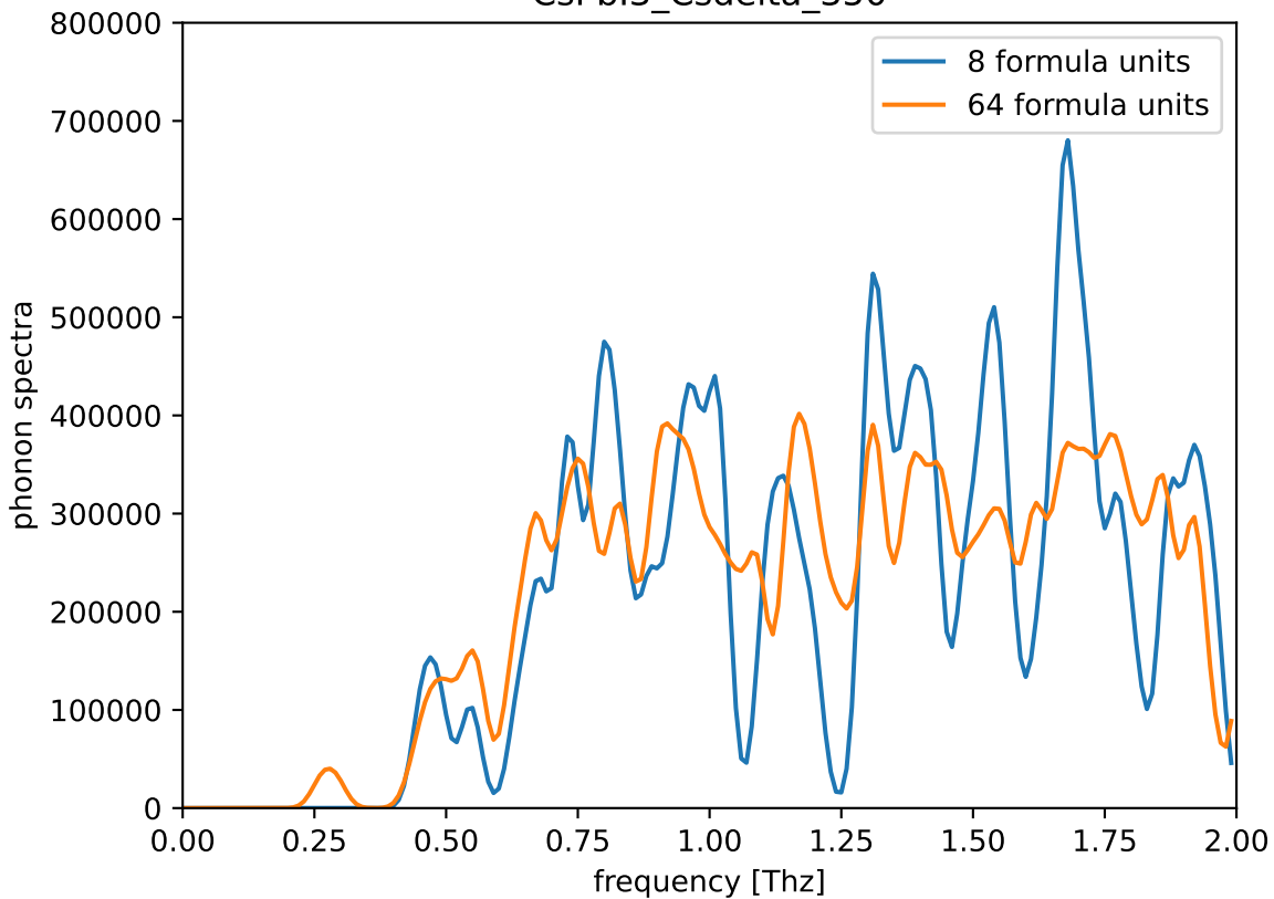
CsPbI3_Csdelta_350
