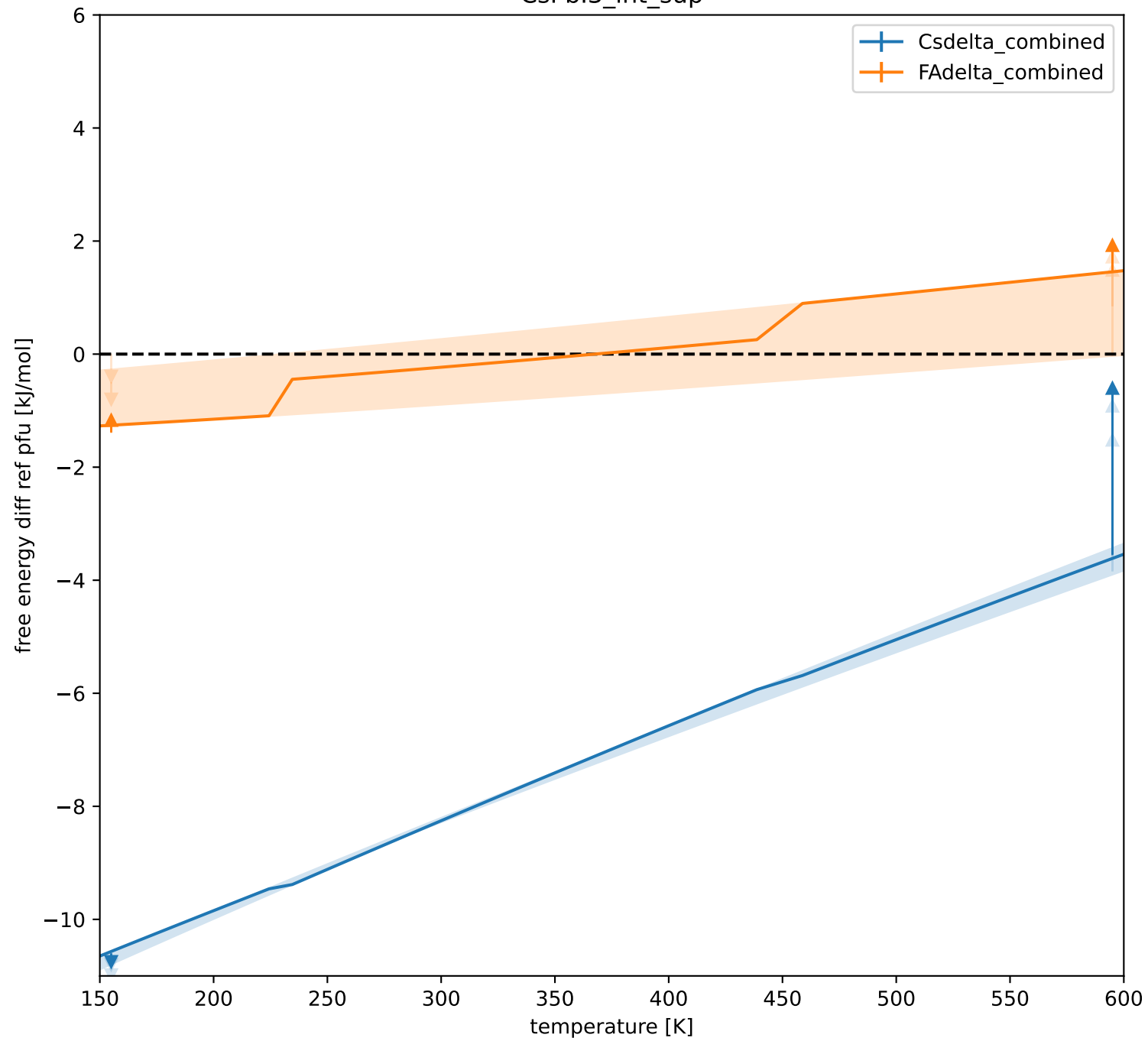
CsPbI3_int_sup
