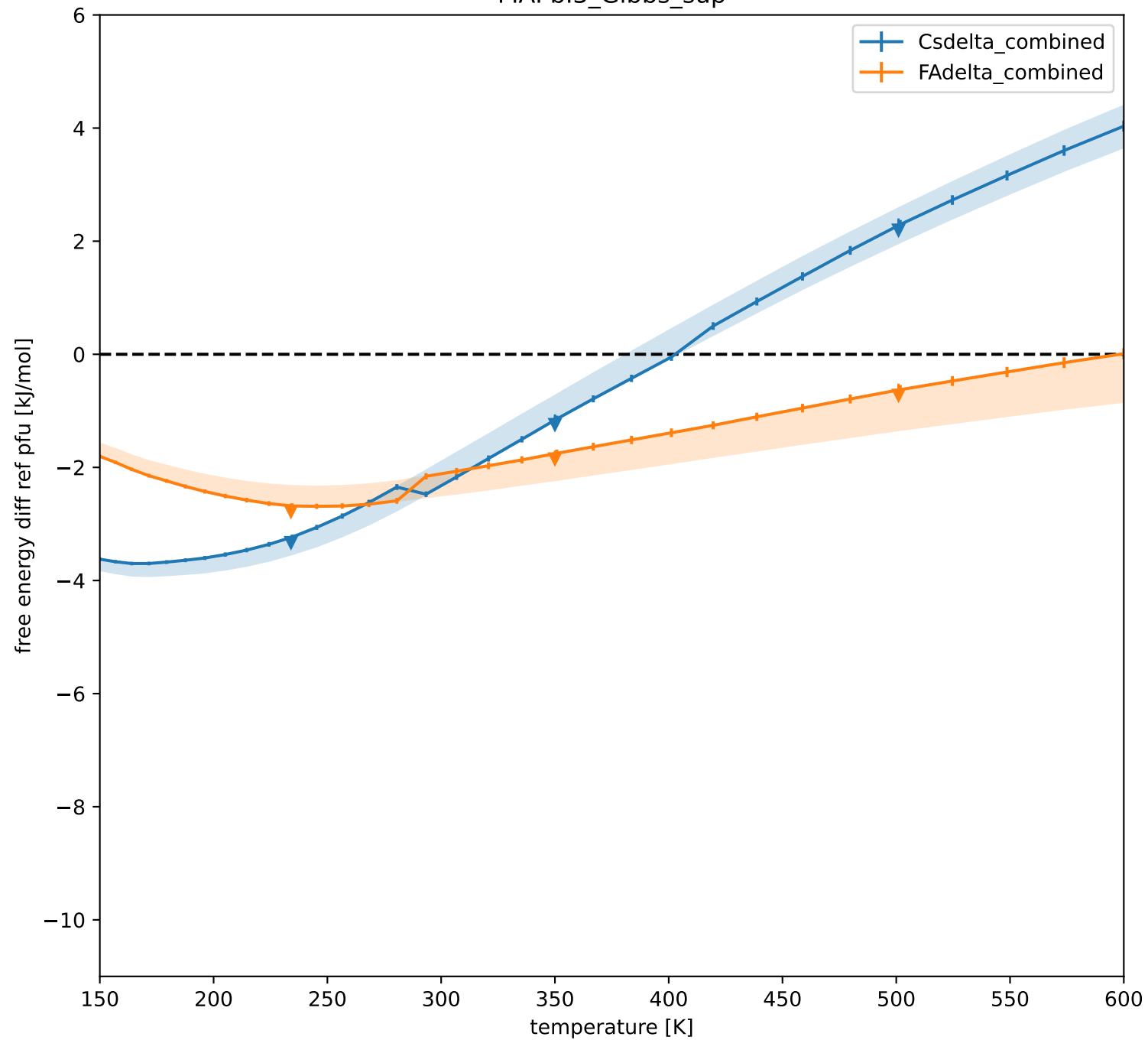
MAPbI3_Gibbs_sup
