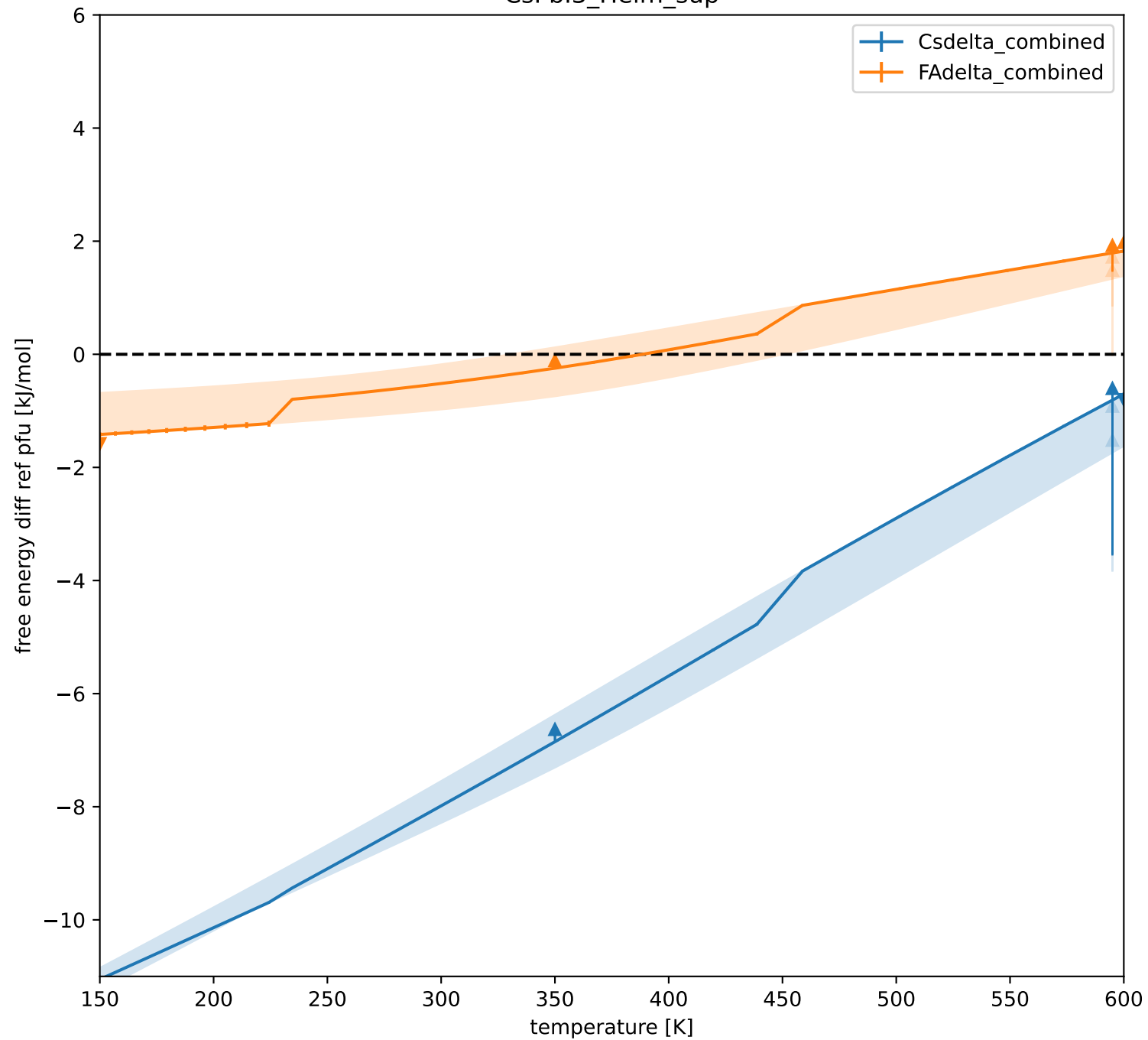
CsPbI3_Helm_sup
