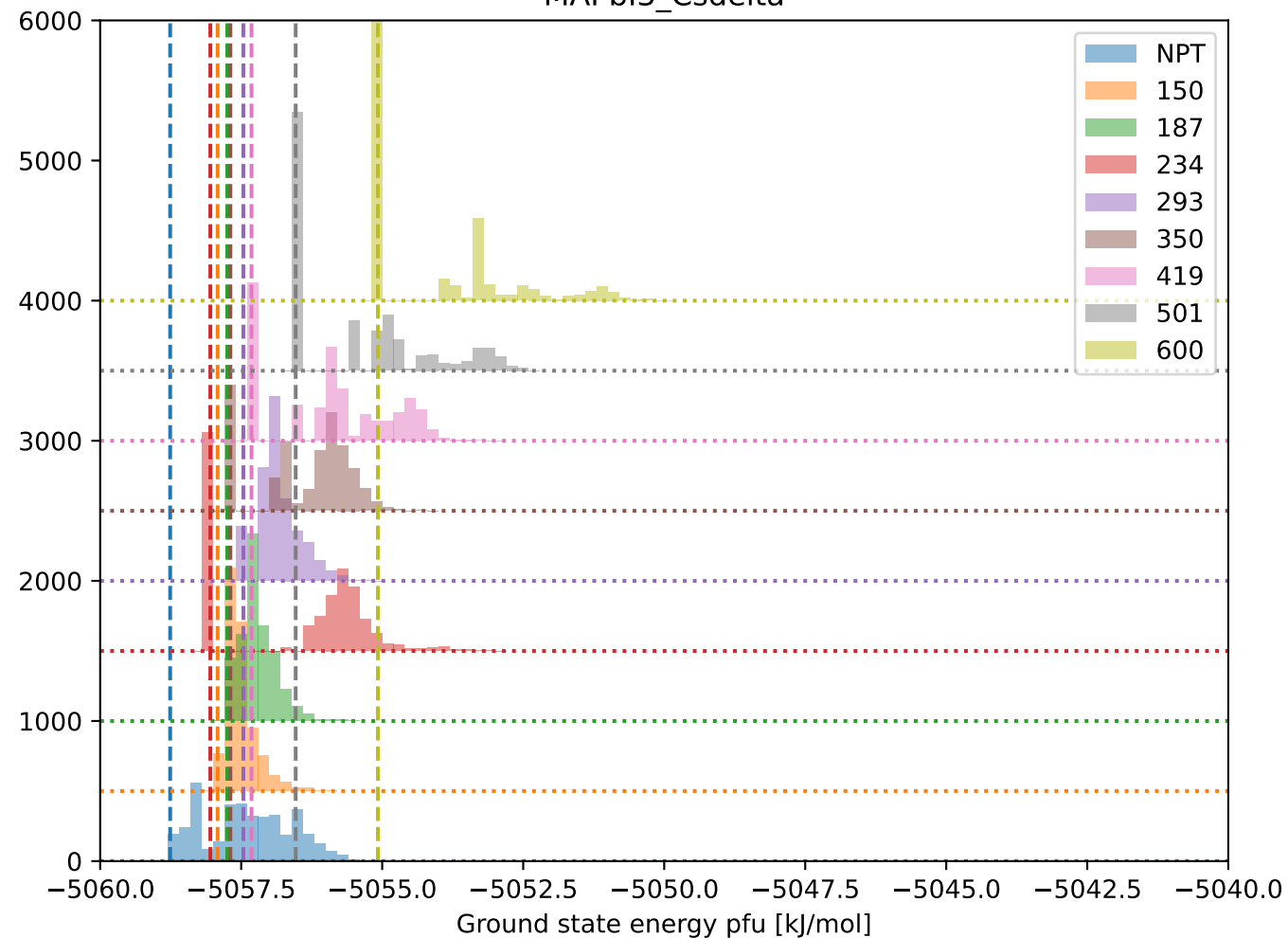
MAPbI3_Csdelta
