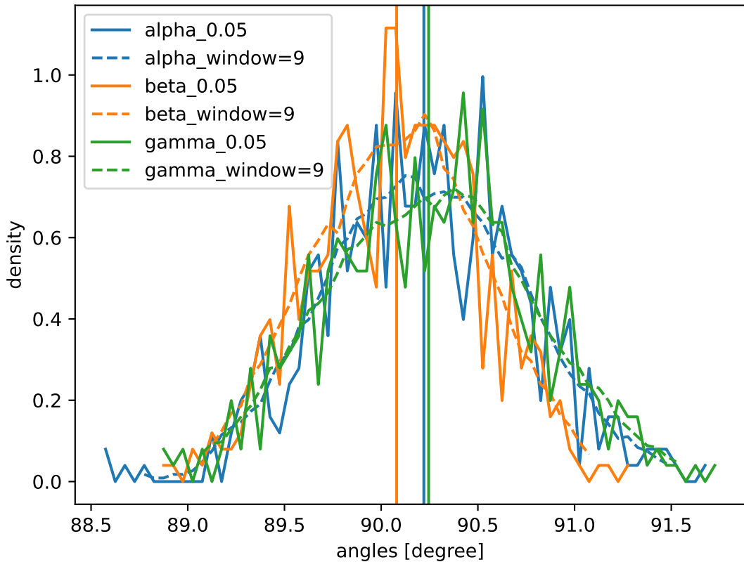
499.0 K, 0.1 MPa
