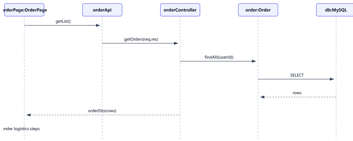
OBJ-SEQ10 订单与物流查询对象调用
