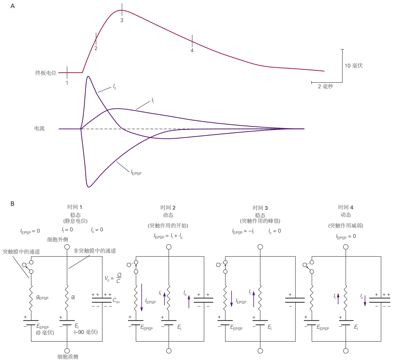
图 12.5.2: 终板电位的时间进程由乙酰胆碱门控突触电导和肌肉细胞的被动膜特性决定。A. 终板电位和通过乙酰胆碱受体通道 ( I_{EPSP} )、静息 (或泄漏) 通道 ( I_l ) 和电容器 ( I_c ) 分量电流的时间过程。只有当膜电位发生变化时才会有电容电流。在稳态下，例如在终板电位的峰值处，通过乙酰胆碱受体通道的内向正电荷流与通过静息通道的外向离子电流完全平衡，并且没有电容电流。B. A 部分所示时间 1、2、3 和 4 电流的等效回路 (电流的相对大小由箭头长度表示)。
