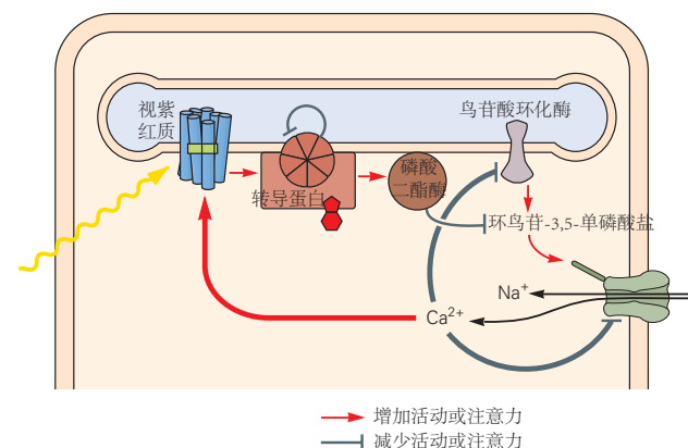
图 22.2.1: 光转导。 A. 视杆细胞对光有响应。外段视盘中的视紫红质分子吸收光子，导致细胞质膜中环鸟苷-3,5-单磷酸盐门控通道关闭。这种通道关闭使膜超极化并降低神经递质谷氨酸的释放速率 [7] 。 B. 1. 光转导中的分子过程。环鸟苷-3,5-单磷酸盐由鸟苷酸环化酶从三磷酸鸟苷产生并被磷酸二酯酶水解。在黑暗中，磷酸二酯酶活性低，环鸟苷-3,5-单磷酸盐浓度高，环鸟苷-3,5-单磷酸盐门控通道开放，允许 \text{Na}^+ 和 \text{Ca}^{2+} 流入。在光线下，视紫红质通过吸收光子而被激发，然后激活转导蛋白，转导蛋白进而激活磷酸二酯酶；环鸟苷-3,5-单磷酸盐水平下降，膜通道关闭，更少的 \text{Na}^+ 和 \text{Ca}^{2+} 进入细胞。转导酶均位于内膜圆盘中，可溶性配体环鸟苷-3,5-单磷酸盐作为细胞质膜的信使。 2. \text{Ca}^{2+} 在光转导响应级联中具有负反馈作用。光对网络的刺激导致环鸟苷-3,5-单磷酸盐门控通道的关闭。这导致细胞内 \text{Ca}^{2+} 浓度下降。因为 \text{Ca}^{2+} 调节至少 3 个级联组分的功能（视紫红质、鸟苷酸环化酶和环鸟苷-3,5-单磷酸盐门控通道） \text{Ca}^{2+} 的下降抵消了光引起的激发。 C. 灵长类视杆细胞和视锥细胞对强度增加的短暂闪光的电压响应。迹线上的数字越高表示光照强度越大（并非所有迹线都已标记）。对于昏暗的闪光，响应幅度随强度线性增加。在高强度下，受体饱和并在闪光后的一段时间内稳定地保持超极化；这会导致我们在明亮的闪光后看到的残像。请注意，对于更亮的闪光，响应峰值更早，并且视锥细胞的响应速度比视杆细胞快 [196] 。
