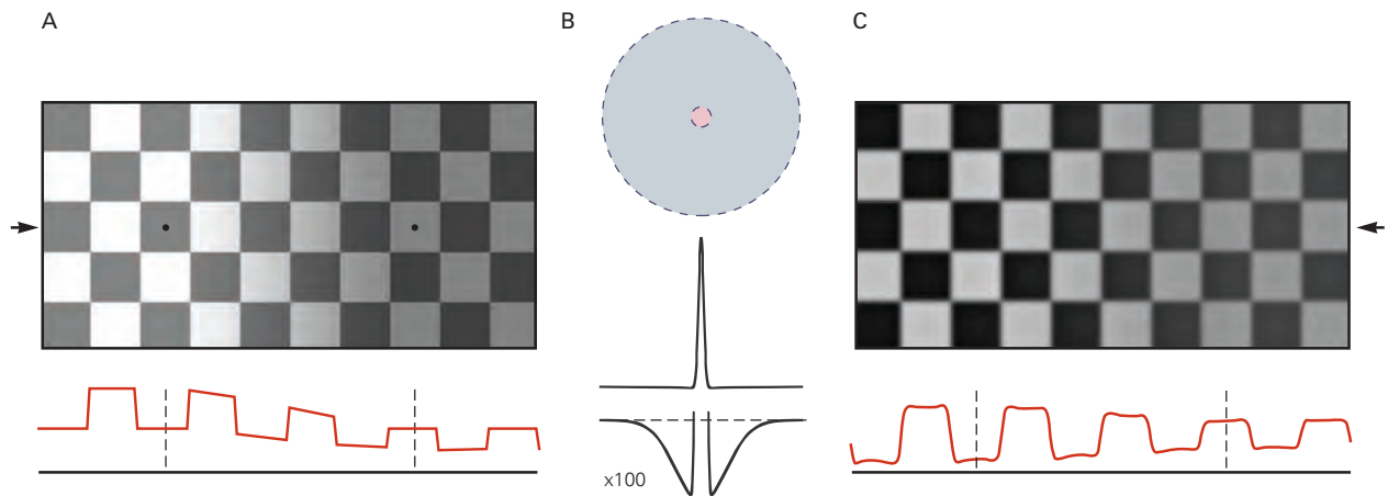
图 22.5.1: 亮度错觉。 A. 标有小点的 2 块瓷砖看起来颜色不同，但实际上反射的光强度相同（要看到这一点，请折叠页面，使它们接触）。下方的迹线绘制了箭头水平的光强度分布图。您的视觉系统将此视网膜图像解释为空间变化照明下的规则图块图案，右半部分有漫射阴影。根据这种解释，右边的瓷砖必须比左边的颜色浅，这就是您所感知的。这个过程是自动的，不需要有意识的分析。B. 视网膜处理通过降低阴影平滑的照明梯度并突出棋盘区域之间的锐利边缘来促进“亮度”的感知。具有兴奋中心和抑制周围的视觉神经元的感受野显示在顶部。如底部放大百倍所示，环绕声较弱，但延伸的区域比中心区域大得多。C. 当一群具有 B 中感受野的视觉神经元处理 A 中的图像时的结果。这个操作（A 中的图像与 B 中的轮廓的卷积）从视野中的每个点中减去大周围区域的平均强度。目标的神经表示在很大程度上失去了阴影的影响，并且所讨论的 2 个图块在该表示中确实具有不同的亮度值。
