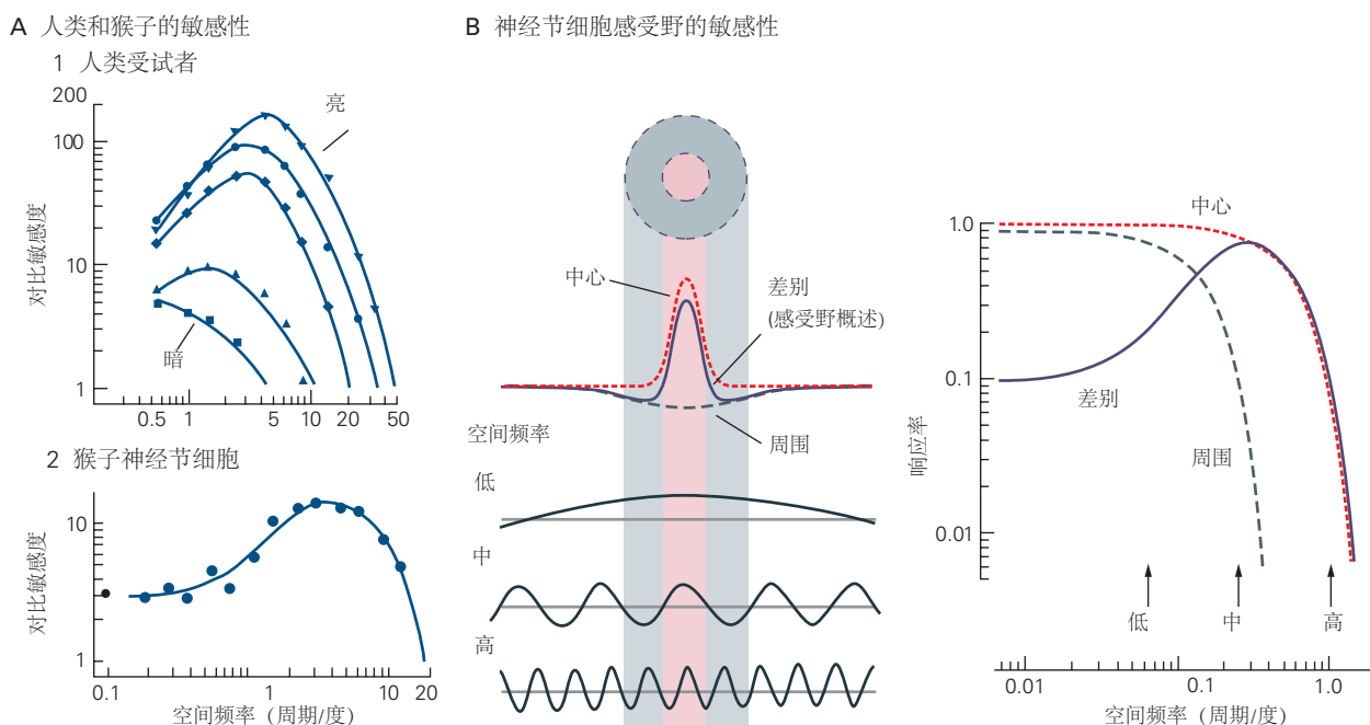
图 22.5.3: 空间对比敏感度。 A. 1. 如图 22.5.4 所示，人类受试者的对比敏感度使用具有不同空间频率的光栅测量。如图所示，在每个频率下，对比度增加到检测阈值，并且该对比度值的倒数相对于空间频率绘制。这些曲线是在不同的平均强度下获得的，从顶部到底部曲线减少了 10 倍 [202] 。2. 在高强度下测量的猕猴视网膜中 P 型神经节细胞的对比敏感度。在每个空间频率下，对比度逐渐增加，直到它在神经元的放电率中产生可检测的变化。如 A-1 部分所示，绘制了该阈值对比度的倒数。左侧的孤立点标记了零空间频率下的灵敏度，这是一个空间均匀的场 [203] 。B. 用正弦光栅刺激中心环绕感受野。神经元对视网膜上不同点的光的敏感性被建模为“高斯差分”感受野，其中兴奋性中心为窄正高斯分布，抑制性周围为宽的负高斯分布。将光栅刺激的轮廓（强度与位置）与感受野的轮廓（灵敏度与位置）相乘，并在所有空间上积分，计算出特定光栅传递的刺激强度。右图显示了感受野对不同频率光栅的灵敏度。在低空间频率下，环绕声的负贡献抵消了中心的贡献，导致差异曲线下降 [204] 。
