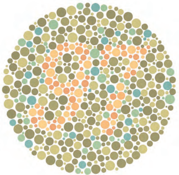
图 22.4.3: 对某些形式的色盲测试。嵌入这种颜色图案中的数字可以被具有三色视觉的人辨别出来，但不能被红绿辨别力较弱的二色视者辨别出来。如果您没有看到任何数字，请检查您的视力。
