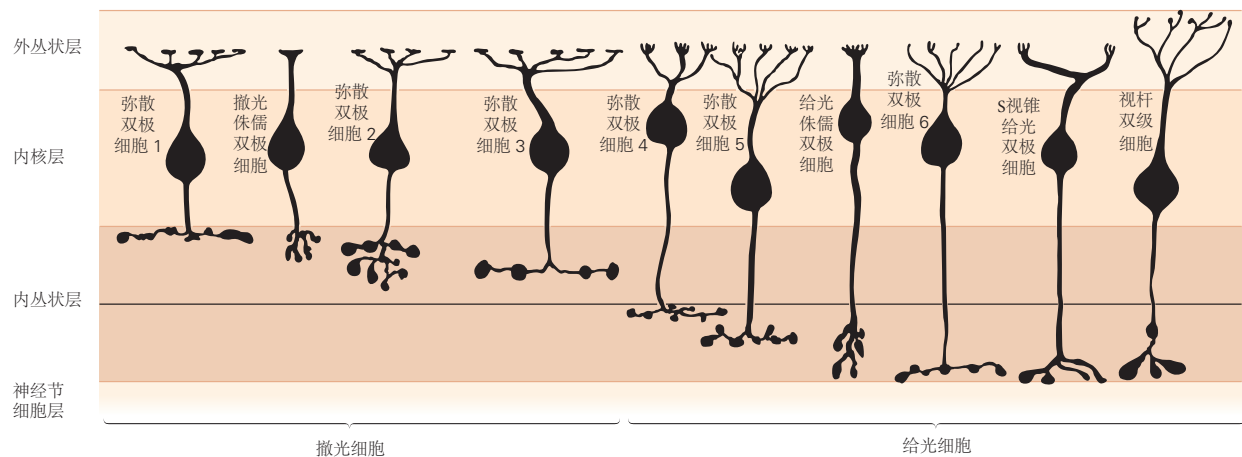
图 22.4.1: 猕猴视网膜中的双极细胞。细胞根据其在内网层中的末端分枝的深度排列。划分该层的远端（上）和近端（下）水平的水平线表示给光型细胞和给光型细胞的轴突末梢之间的边界。假定上半部分的端子是 给光细胞的端子，下半部分的端子是给光单元的端子。细胞类型是弥散双极细胞、给光小型双极细胞和给光小型双极细胞、短波锥双极细胞和杆状双极细胞。
