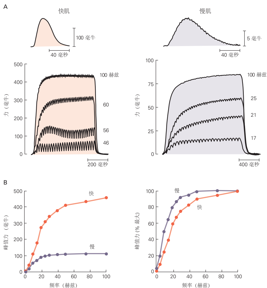
图 31.1.2: 运动单位施加的力随其神经元产生动作电位的速率而变化。A. 轨迹显示快速和慢速收缩运动单位响应单个动作电位（顶部轨迹）和一系列动作电位（下面的 4 个轨迹组）所施加的力。速度更快的单元达到峰值抽搐力或收缩时间的时间更短。用于引起强直性收缩的动作电位的速率范围从慢速收缩单元中的 17 到 100 赫兹到快速收缩单元中的 46 到 100 赫兹。由 100 赫兹刺激引起的强直力峰值对于快速收缩单元来说更大。注意 2 组迹线的不同力标度 [278-280] 。B. 快速收缩和慢速收缩运动单位的峰值力和动作电位之间的关系。在所有频率下，快速收缩的运动单位的绝对力（左图）都更大。在较低的刺激率下（右图），与快速收缩的运动单位（较短的收缩时间）相比，慢速收缩的运动单位（较长的收缩时间）产生的相对力（峰值力的百分比）更大。
