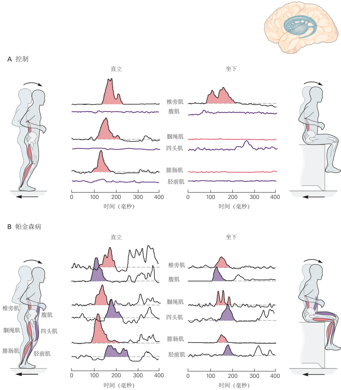
图 36.5.3: 基底神经节对于适应初始条件突然变化的姿态响应很重要 [361] 。A. 当正常受试者从直立姿态转换为坐姿时，他会立即改变对支撑平台向后移动的响应。坐着时对运动的姿态响应不涉及腿部肌肉（腓肠肌和腓绳肌），但会激活椎旁肌，并且比站立时对运动的响应延迟更短。B. 帕金森病患者在从站立转为坐姿后的第一次试验中没有抑制腿部肌肉响应。该受试者的姿态响应对于 2 个初始位置都相似：拮抗肌（紫色）与激动肌（粉红色）一起被激活。
