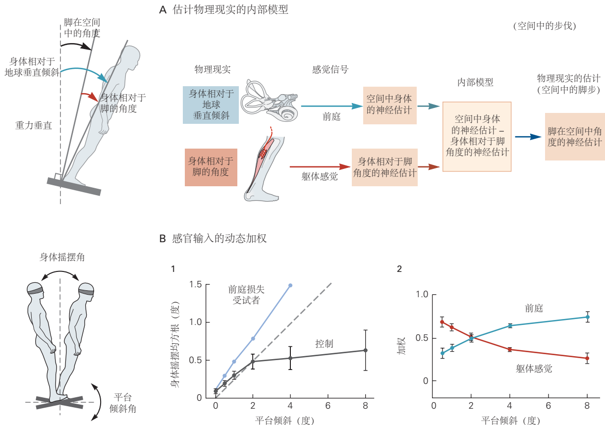
图 36.3.4: 许多类型的感官信号在优化平衡和方向的内部模型中被集成和加权 [358] 。A. 一个人站在倾斜的表面上简单例子说明了神经系统如何估计无法直接感知的物理变量。物理变量是身体相对于地球垂直倾斜，以及身体相对于脚的角度。脚在空间中的角度就是差值身体相对于地球垂直倾斜 - 身体相对于脚的角度。空间中身体的神经估计来自前庭和其他检测身体相对于重力倾斜的受体。身体相对于脚角度的神经估计来自与踝关节角度相关的体感信号。用于估计物理现实的内部模型空间中身体的神经估计 - 身体相对于脚角度的神经估计产生脚在空间中角度的神经估计。这种对物理世界的估计会根据经验不断更新。B. 感官信息动态加权以在不同条件下保持平衡和定向。该图说明了一项实验的结果，在该实验中，人类受试者蒙着眼睛站在一个平台上，该平台以高达 8°（峰到峰）的幅度在脚趾向上或脚趾向下的方向上连续缓慢旋转。1. 前庭功能丧失的受试者和一组对照受试者在表面振荡期间身体摇摆的比较。车身摇摆角是在平台倾斜期间相对于重力垂直方向测量的，并表示为以度为单位的均方根摇摆。虚线代表平等的平台和身体摇摆；例如，对于 4° 的平台倾斜，等量的身体摇摆是 1° 均方根。在控制对象中，身体和平台的摇摆对于小平台倾斜高达 2° 是相等的，这表明人们通常使用体感信号来保持与平台的垂直（最小化脚踝角度的变化）。对于更大的平台倾斜度，车身摇摆不会增加太多超过 0.5° 均方根。相比之下，前庭功能丧失的受试者比平台摇摆得更多（平台倾斜度为 4° 时身体倾斜度为 1.5° 均方根）并且不能在平台倾斜度超过 4° 时保持站立。因此，当前庭信号和视觉信号均不存在时，人试图仅相对于支撑表面保持其位置并且难以在该表面移动时保持平衡。2. 在控制对象中，随着平台倾斜度的增加，体感输入的影响随着平台倾斜度的增加而减小，而前庭输入的影响增加。在更大的倾斜角度下，前庭输入的影响更大，可以最大限度地减少身体偏离重力垂直方向的程度。
