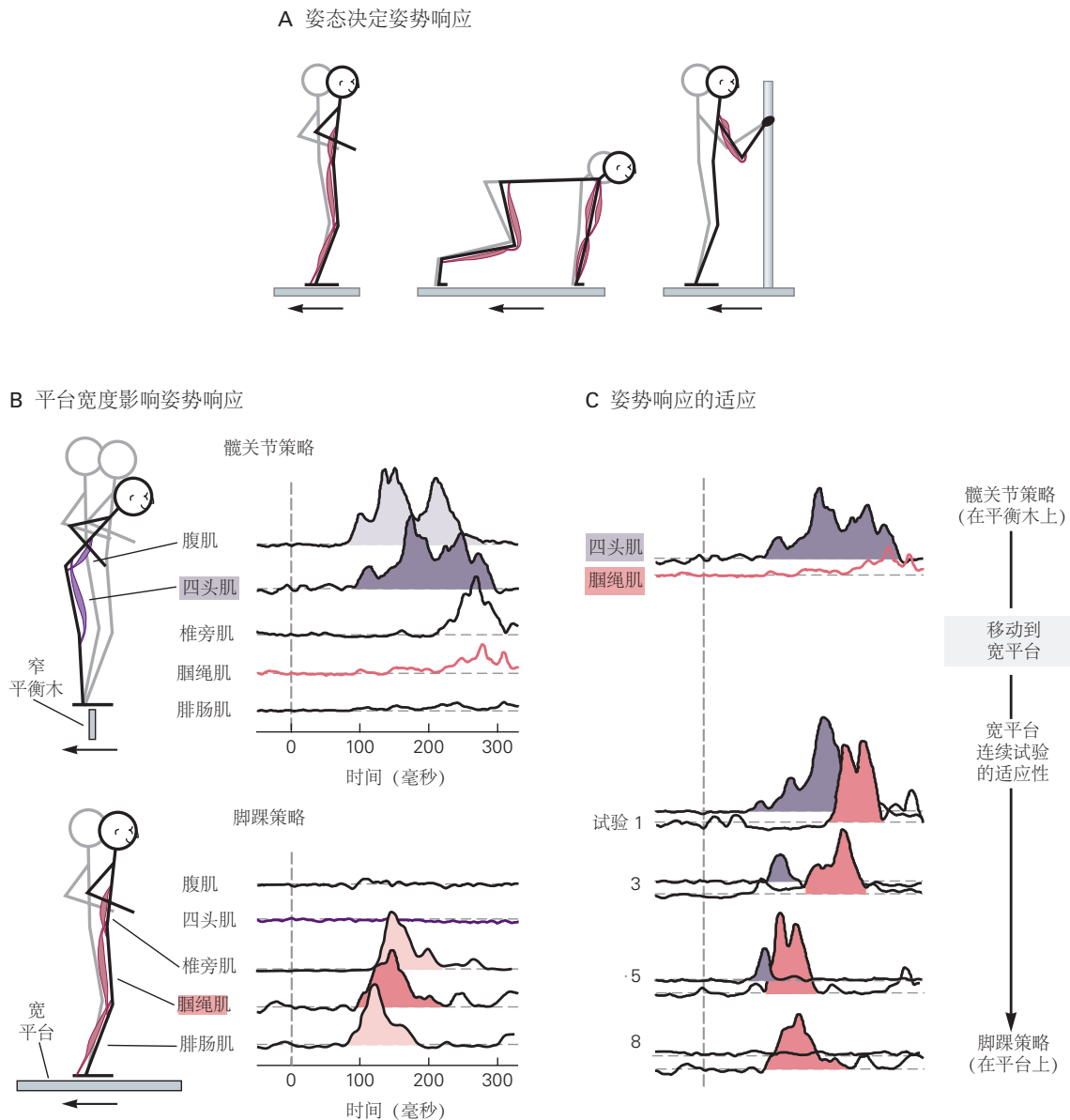
图 36.2.5: 自动姿态响应随生物力学条件而变化。A. 平台的向后运动会根据初始姿态激活不同的肌肉群。灰色简笔画显示初始位置（无支撑直立、四足支撑或直立支撑）。在每个姿态响应中激活的肌肉以红色显示 [352] 。B. 当受试者站在一根突然向后移动的窄平衡木上时，前部肌肉（腹肌和四头肌）被募集来弯曲躯干，并伸展脚踝，向后移动髋关节（髋关节策略）。当受试者站在一个向后移动的宽平台上时，他的后部肌肉（椎旁肌、腓绳肌和腓肠肌）会被激活，通过旋转脚踝使身体恢复直立姿态（脚踝策略）。代表不同姿态响应的肌肉以颜色突出显示。图中的垂直虚线表示平台（或平衡木）加速的开始。C. 受试者从窄平衡木移动到宽平台后姿态策略适应。在平衡木上，股四头肌被激活，腓绳肌沉默；适应宽平台后，观察到相反的情况。从股四头肌到腓绳肌激活的转变发生在一系列试验中；股四头肌的活动幅度逐渐减小，而腓绳肌被激活的时间越来越早，直到试验 8，股四头肌的活动完全消失。脚踝和躯干肌肉表现出相似的适应模式 [353] 。
