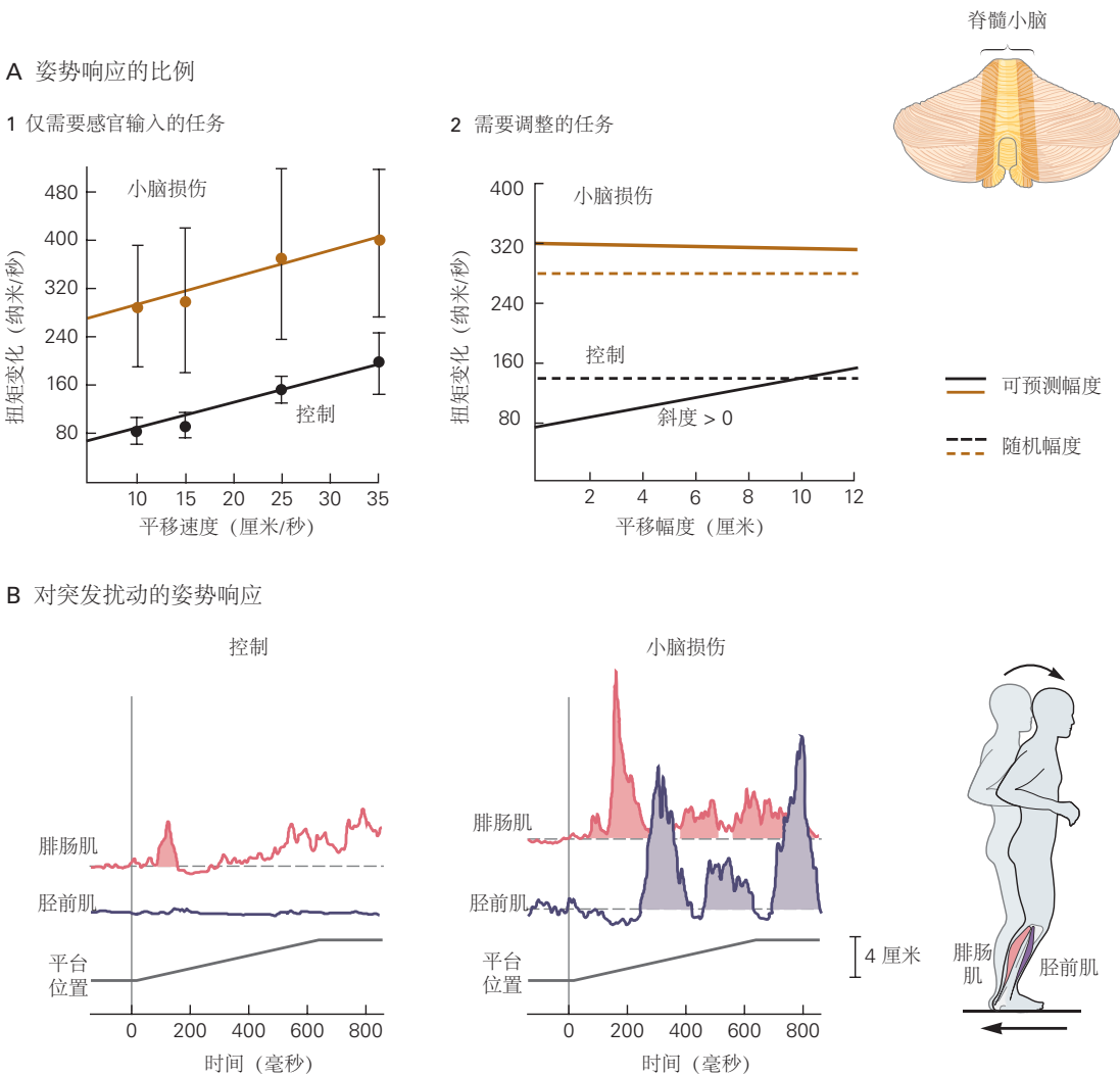
图 36.5.2: 脊髓小脑在适应不断变化的条件的姿态响应和调整对预期姿态障碍的姿态响应方面发挥作用。脊髓小脑对于根据经验调整姿态响应很重要。脊髓小脑疾病患者能够使用即时感觉输入，但不能使用经验来调整自动姿态响应 [360] 。A. 1. 在这个实验中，受试者站在一个水平移动的平台；每次试验都会增加速度。保持平衡需要使用感官反馈来缩放对平台速度的响应。患有脊髓小脑疾病的受试者的调整具有与对照受试者相同的回归系数（斜率），即使在每个试验中的响应比对照受试者的响应更大且变化更大。2. 当受试者需要预测和适应平台平移时，脊髓小脑受试者的姿态调整就会受到影响。当平移幅度是随机的时，响应很大，就好像受试者期望一个大的平移一样。当重复相同振幅的试验时，控制对象学会预测干扰的振幅并调整他的响应。相比之下，脊髓小脑受试者的表现没有任何改善；他不能利用他在一次试验中的经验来调整他在随后试验中的响应。所有的回复都很大，就好像受试者总是期待大的翻译。B. 在此实验中，受试者站在向后移动的平台（6 厘米振幅，10 厘米/秒）。在对照对象中，运动的开始会引起腓肠肌（一种踝关节伸肌）的小幅活动爆发。在小脑前叶受损的受试者中，肌肉响应过大，胫前肌及其拮抗剂腓肠肌之间交替出现爆发性活动。
