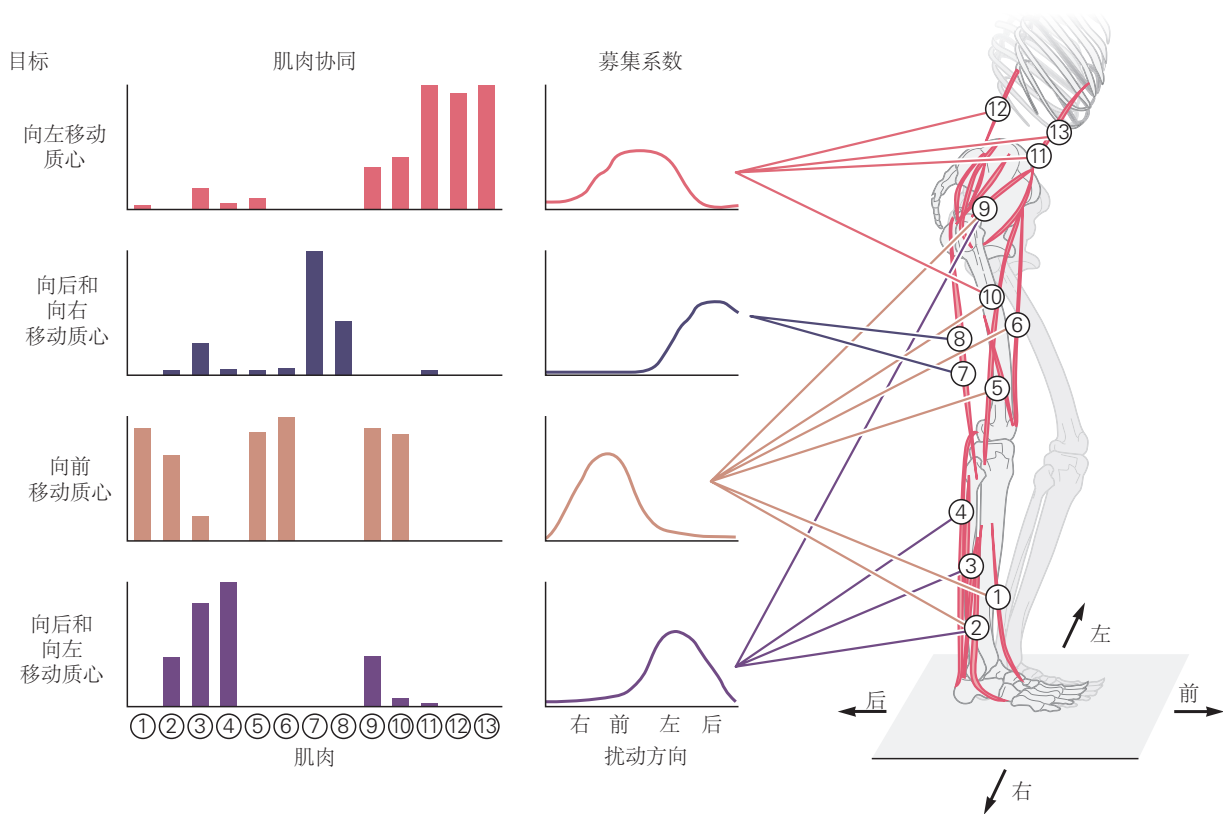
图 36.2.4: 姿态指令激活协同效应，而不是单个肌肉。几个肌肉的协同激活可以将运动目标转化为特定的肌肉激活模式。每一种肌肉协同作用都会以固定的比例激活一组肌肉（彩色条），以产生实现姿态目标所需的机械输出。每个小节的高度代表每个肌肉的相对激活量或权重（1-13）。在由中央命令和感觉驱动（募集功能）驱动的行为过程中，每一种协同作用或多或少在特定时间被激活。例如，不同的姿态协同作用在不同的跌倒方向上被激活。
