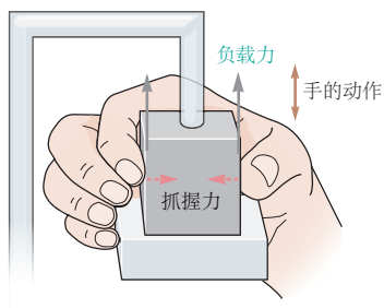
图 30.4.5: 对自发动作的超前控制 [272] 。A. 当指示受试者握住以机械方式施加正弦负载力的物体时，手指的抓握力很高以防止滑动，并且抓握力调节滞后于负载力的变化。其中以深红色实线突出显示的是负载力调节的一部分，这会导致深红色虚线所示的相应抓握力滞后（试验时长为 4 秒）。B. 当受试者通过下拉固定物体产生类似的负载曲线时，可以预期负载力，因此，抓握力较低并且跟踪负载力没有延迟。
