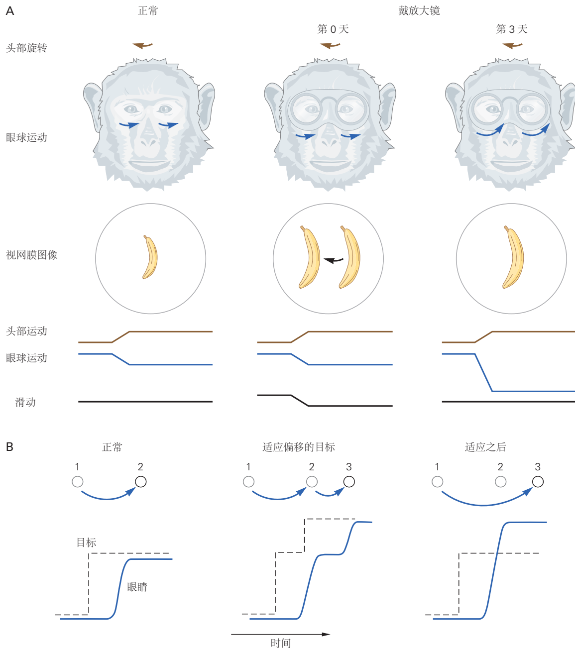
图 37.5.3: 前庭-眼动反射和眼跳中的小脑学习。A. 戴着放大镜的猴子前庭-眼动反射的运动学习。这些列显示了学习前的正常情况，猴子第一次戴眼镜时的情况（第0天），以及完全适应后的情况（第3天）。眼睛的运动通常与转头相等且相反，在转头过程中香蕉在视网膜中保持稳定。戴上眼镜，香蕉看起来更大了；当头部转动时，前庭-眼动反射太小，香蕉的图像滑过视网膜。适应后，眼睛的运动足够大，以至于在转头时香蕉的图像在视网膜上再次保持稳定 [371] 。B. 眼跳中的运动学习。这些列显示了在正常条件下、第一次适应试验和完全适应后的眼跳。通常，眼跳通过将眼睛几乎完美地带到新的目标位置来响应目标位置的变化。在适应过程中，目标在初始眼跳过程中移动到新的位置，需要第二次眼跳才能将眼睛带到新的最终目标位置。在适应之后，原始目标位置唤起更大的眼跳，即使目标没有移动，也适合将眼睛带到新的目标位置。
