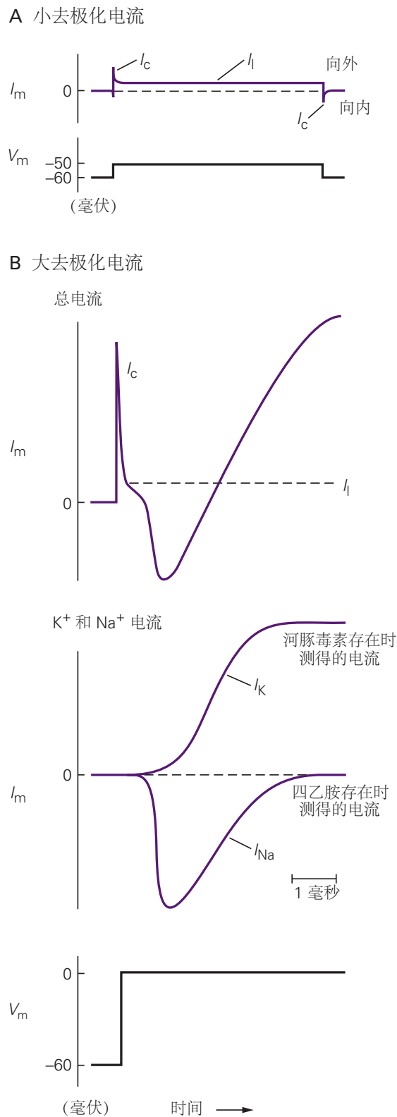
图 10.1.3: 电压钳实验演示了电压门控 Na + 通道和 K + 通道的顺序激活。A. 小的去极化 (10 毫伏) 会引发电容电流 I_c 和漏电流 I_l ，它们是总膜电流 ( I_m ) 的组成部分。B. 较大的去极化 (60 毫伏) 会导致较大的电容电流和漏电流，以及随时间变化的内向离子电流和随时间变化的外向离子电流。顶部：响应去极化的总 (净) 电流。中间：单独的 Na + 电流和 K + 电流。在存在阻断 Na + 电流的河豚毒素或存在阻断 K + 电流的四乙胺的情况下使细胞去极化，显示减去后的纯 K + 和 Na + 电流 (分别为 I_K 和 I_{Na} ) I_c 和 I_l 。底部：电压阶跃。
