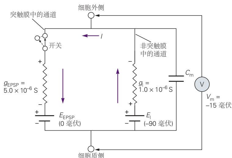
图 12.5.1: 终板的等效回路。该回路具有 3 个平行的电流。一种电导通路承载终板电流，由串联的乙酰胆碱受体在突触后膜上产生的电位差与乙酰胆碱受体 ( g_{EPSP} ) 的电导 ( E_{EPSP} ) 组成。另一个电导路径通过非突触膜传输电流，由代表静息电位 ( E_I ) 的细胞静息电位与静息通道的电导 ( g_I ) 串联组成。与这两条电导通路并联的是膜电容 ( C_m )。电压表 (V) 测量细胞内外之间的电位差。当不存在乙酰胆碱时，乙酰胆碱受体通道关闭并且不传导电流。这种状态被描述为一个开式的回路，在这个回路中，突触电导没有连接到回路的其余部分。乙酰胆碱的结合打开突触通道。此事件在电气上等效于打开连接门控电导通路 ( g_{EPSP} ) 与静息通路 ( g_I ) 的开关。在稳定状态下，通过乙酰胆碱受体通道的内向电流与通过静息通道的外向电流平衡。根据所示的电导值和电池值，膜将从 -90 毫伏（其静息电位）去极化至 -15 毫伏（终板电位的峰值）。
