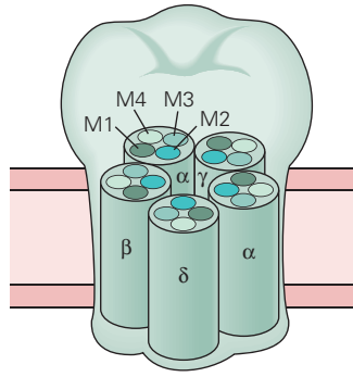
B 通道孔周围亚基的排列
