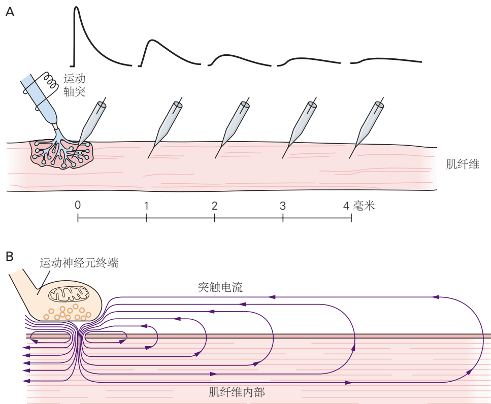
图 12.1.3: 终板电位随着它被动的从终板处传播开去，振幅随距离减少。A. 突触后电位的振幅减小，并且电位的时间进程随距离离开起始点而减慢。B. 这种衰减是由于肌肉纤维膜的泄漏导致的。因为电荷必须在一个完整的回路中流动，所以终板处的内向突触电流会通过静息通道和脂质双层（即电容器）产生返回的外向电流。这种返回的正电荷向外流动使膜去极化。因为电流沿着膜一直漏出，所以向外的电流和由此产生的去极化会随着与终板的距离的增加而减小。
