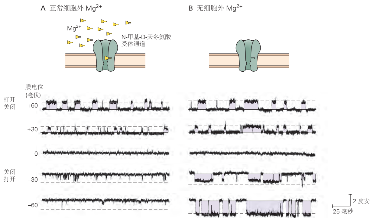
图 13.3.6: 除了谷氨酸之外，单个 N-甲基-D-天冬氨酸受体通道的打开还取决于膜电位。这些膜片钳记录来自单个 N-甲基-D-天冬氨酸受体通道（来自培养的大鼠海马细胞）。向下偏转表示内向（负）电流脉冲；向上偏转表示外向（正）电流。 A. 当 Mg^{2+} 以正常浓度存在于细胞外溶液（1.2 毫摩尔）时，该通道在静息电位（-60 毫伏）处大部分被阻断。在负膜电位下，由于 Mg^{2+} 阻滞，在通道打开时只能看到短暂、闪烁的内向电流。对 0 毫伏反转电位（至 +30 毫伏或 +60 毫伏）正电压的大量去极化解除了 Mg^{2+} 阻滞，允许更持久的外向电流脉冲通过通道。 B. 当 Mg^{2+} 从细胞外溶液中去掉时，通道的打开和关闭不依赖于电压。如图 13.3.7B 所示，通道在 -60 毫伏的静息电位下打开，突触电流在接近 0 毫伏时反转，就像总突触电流一样。
