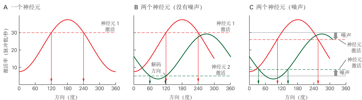
图 39.2.2: 准确的运动解码需要不止一个神经元。A. 一个神经元的调谐曲线定义了神经元的活动如何随运动方向变化。如果此神经元显示 30 个脉冲/秒的活动，则它可能对应于 120° 或 240° 方向的运动。B. 具有不同调谐曲线的第二个神经元（绿色）显示 5 个脉冲/秒的活动，这可能对应于 60° 或 120° 方向的运动。唯一与 2 个神经元的活动一致的运动方向是 120°，这被确定为解码方向。C. 因为神经活动是“嘈杂的”（表示为虚线的垂直位移），通常不可能从 2 个神经元的活动中最终确定运动方向。在这里，没有一个运动方向与 2 个神经元的活动一致。
