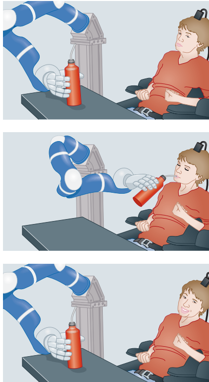
图 39.3.3: 一名瘫痪的受试者使用机械臂从瓶子里喝水，机械臂由使用连续解码器的运动脑机接口控制。第一次成功试验的三张连续图像显示，受试者使用机械臂抓住瓶子，把它放到嘴里，用吸管喝咖啡，然后把瓶子放回桌子上 [379] 。
