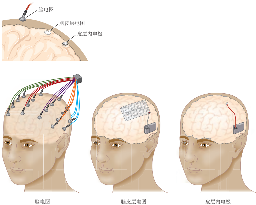
图 39.1.2: 脑机接口使用不同类型的神经传感器。可以使用各种技术测量电神经信号，从皮肤表面的脑电图电极到大脑表面的脑皮层电图电极，再到植入皮层外 1 至 2 毫米的皮层内电极。可以测量的信号范围从许多神经元的平均值到较少神经元的平均值，最后到单个神经元的动作电位 [375] 。
