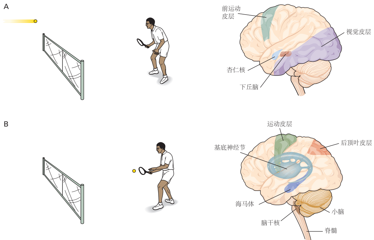
图 4.1.2: 一个简单的行为由大脑的许多部分调节。 A. 一名网球运动员在观看接近的球时使用视觉皮层来判断球的大小、方向和速度。而前运动皮层则会制定出一个动作程序以回应击球。与此同时，杏仁核与其他大脑区域协作，调节心率、呼吸和其他内稳态机制，并激活下丘脑，激发选手击球的良好动机。 B. 要完成这一击球动作，选手必须动用 A 部分中提到的所有结构，以及其他一些结构。运动皮层向脊髓发出信号，激活和抑制手臂和腿部的许多肌肉。基底神经节开始参与启动运动模式，并可能回忆起学习的动作以正确击球。小脑根据来自外周感觉受体的本体感受信息调整运动。后顶叶皮层给予选手空间定位感，让他知道自己身体在空间中的位置以及球拍相对于身体的位置。脑干神经元在整个动作过程中调节心率、呼吸和唤醒水平。海马体并不直接参与击球过程，但它参与存储这次击球的记忆，以便选手稍后可以夸耀此事。
