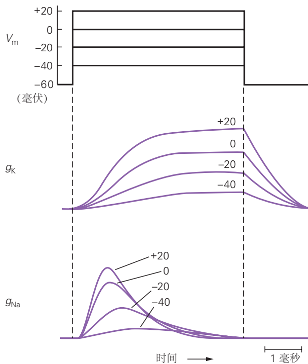
图 10.1.6: K^+ 通道和 Na^+ 通道对长时间去极化的响应。增加去极化引起 K^+ 电导 g_K 和 Na^+ 电导 g_{Na} 的分级增加，这反映了数千个电压门控 K^+ 和 Na^+ 通道的比例开放。 Na^+ 通道比 K^+ 通道打开得更快。在维持去极化过程中，由于失活门的关闭， Na^+ 通道在打开后关闭。 K^+ 通道保持开放状态是因为它们缺乏快速灭活过程。在非常正的 V_m 下， K^+ 和 Na^+ 电导接近最大值，因为去极化足以打开几乎所有可用通道。
