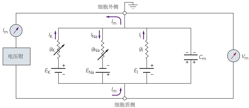
图 10.1.5: 电压钳神经元的等效回路。电压门控电导通路（ g_K 和 g_{Na} ）用可变电导的符号表示，即带有箭头的导体（电阻器）。电导是可变的，因为它依赖于时间和电压。这些电导与代表 Na^+ 和 K^+ 化学梯度的细胞串联。此外，泄漏电流（ g_l 和 E_l ）和电容电流（ C_m ）也有并行的通路。箭头表示激活 g_K 和 g_{Na} 的去极化步骤中的电流。
