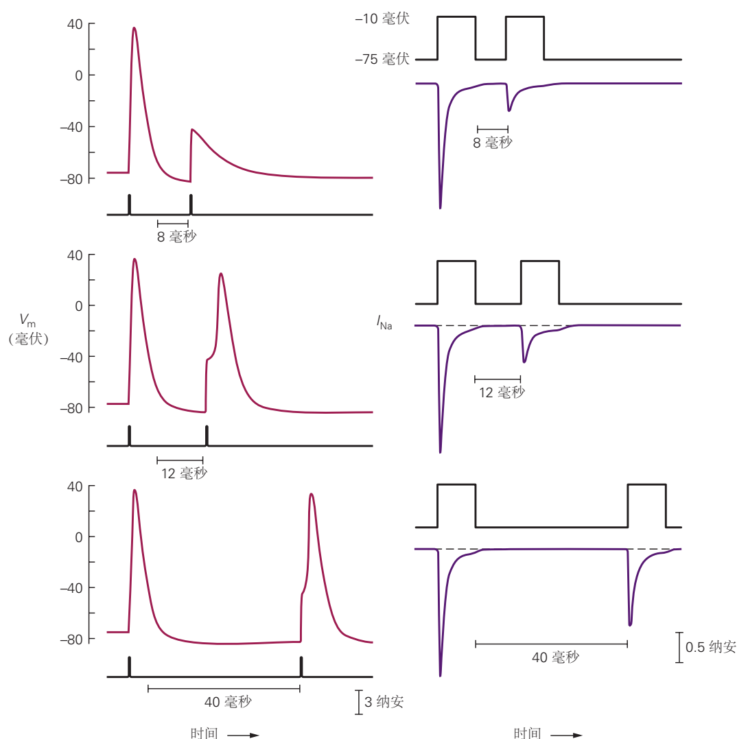
图 10.1.8: 不应期与 Na^+ 通道从失活中恢复有关。左图：小鼠背根神经节神经元对 2 个电流脉冲的电压响应（底部迹线）。第一个触发动作电位；第二个触发可变电压响应，具体取决于电流脉冲之间的延迟。右图：由 2 个去极化电压脉冲引起的同一个细胞在电压钳下记录的钠电流，2 个去极化电压脉冲由左侧记录中指示的间隔分开。在这个神经元中，不应期对应于恢复大约 20% 的 Na^+ 通道所需的时间。
