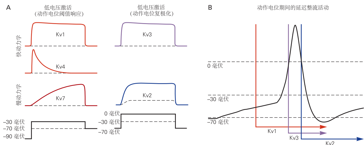
图 10.4.3: 哺乳动物电压激活 K + 通道主要类别的不同电压门控和动力学。A. 主要电压门控 K + 家族的电压门控和动力学的简化概括。由于 Kv1、Kv4 和 Kv7 通道可以被相对较小的去极化激活，因此它们通常有助于控制动作电位阈值。Kv2 和 Kv3 通道需要更大的去极化才能被激活。Kv1、Kv3 和 Kv4 通道的激活速度相对较快，而 Kv7 和 Kv2 通道的激活速度较慢。B. 动作电位期间延迟整流 K + 通道主要成分的不同激活时间的简化概括。Kv1 通道需要小的去极化并且被迅速激活，有时甚至比动作电位显著提前。Kv3 通道需要大的去极化，并且在动作电位的上升阶段后期被激活，此后非常迅速失活。Kv2 通道在动作电位下降阶段相对缓慢地被激活，并在后超极化期间保持开放 [59] 。
