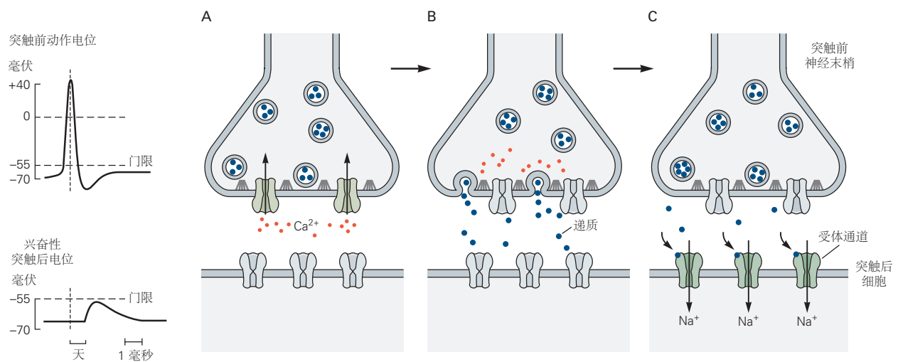
图 11.2.2: 化学突触的突触传递涉及几个步骤。如图 11.2.1B 所示，与电突触处几乎瞬时的信号传递相比，化学突触传递的复杂过程解释了突触前细胞中的动作电位与突触后细胞中的突触电位之间的延迟。A. 到达突触前轴突末梢的动作电位导致活动区的电压门控 \text{Ca}^{2+} 通道打开。灰色细丝代表活性区的对接和释放位点。B. \text{Ca}^{2+} 通道开放在活性区附近产生高浓度的细胞内 \text{Ca}^{2+} ，导致含有神经递质的囊泡与突触前细胞膜融合并将其内容物释放到突触间隙（称为胞吐作用的过程）。C. 释放的神经递质分子然后扩散到突触间隙并结合突触后膜上的特定受体。这些受体导致离子通道打开（或关闭），从而改变突触后细胞的膜电导和膜电位。
