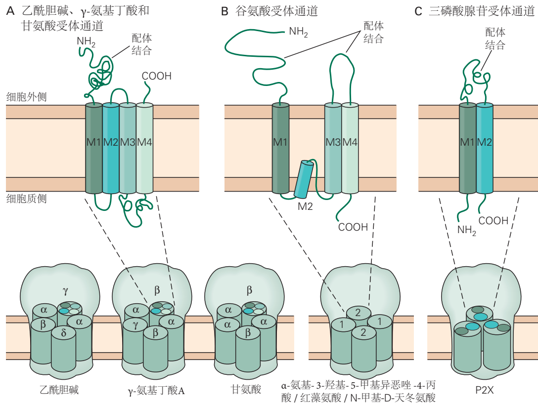
图 13.3.2: 离子型受体的 3 个家族。A. 烟碱乙酰胆碱、 \gamma 氨基丁酸 A 和甘氨酸受体通道都是由几种类型的相关亚基组成的五聚体。如此处所示，配体结合域由蛋白质的细胞外氨基末端区域形成。每个亚基都有 1 个膜结构域，具有 4 个跨膜 \alpha -螺旋（M1-M4）和 1 个短的细胞外羧基末端。M2 螺旋排列通道孔。B. 谷氨酸受体通道是四聚体，通常由 2 种不同类型的密切相关的亚基（此处表示为 1 和 2）组成。这些亚基具有一个大的细胞外氨基末端、1 个具有 3 个跨膜 \alpha 螺旋（M1、M3 和 M4）的膜结构域、1 个连接 M3 和 M4 螺旋的大细胞外环以及一个细胞内羧基末端。M2 部分形成一个环，浸入和浸出膜的细胞质侧，有助于通道的选择性过滤器。谷氨酸结合位点由细胞外氨基末端和 M3-M4 细胞外环中的残基形成。C. 三磷酸腺苷受体通道（或嘌呤 P2X 受体）是三聚体。每个亚基都具有 2 个跨膜 \alpha 螺旋（M1 和 M2）和 1 个结合三磷酸腺苷的大细胞外环。M2 螺旋排列在孔隙中。
