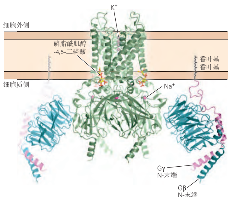
图 14.5.3: G 蛋白 \beta\gamma 亚基可直接结合并激活 G 蛋白门控的内向整流钾通道。G 蛋白门控的内向整流钾通道(绿色)与 G 蛋白 \beta -亚基( G\beta , 青色)和 \gamma -亚基( G\gamma , 紫色)相互作用的高分辨率结构。香叶基香叶基脂质分子连接到 G\gamma 的 C 末端。该结构说明 \text{Na}^+ 和磷脂酰肌醇-4,5-二磷酸也与通道结合,从而增强通道开放。通道内的粉红色球体代表 \text{K}^+ [85] 。
