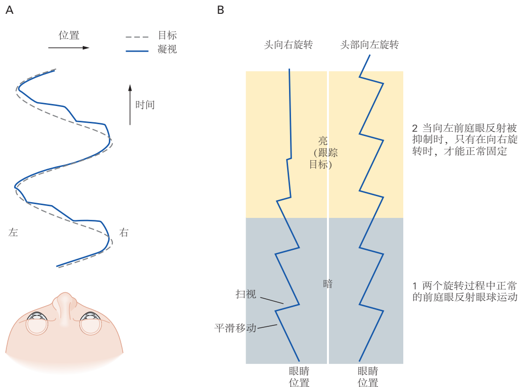
图 37.2.5: 前庭小脑的病变对平滑跟踪眼球运动有很大影响。A. 当目标从左移动到右时, 正弦曲线目标运动通过平滑跟踪眼球运动进行跟踪。由于左侧前庭小脑的损伤, 当目标从右向左移动时, 平滑跟踪会被眼跳打断。B. 在同一名患者中, 对前庭刺激的反应是正常的, 而在向左旋转期间物体固定被打乱。左侧和右侧的痕迹显示了在不同的会话中经历的向右和向左的头部旋转引起的眼球运动。在每次治疗中, 患者坐在一张不断向一个方向旋转的椅子上, 先是在黑暗中, 然后是在光线中, 同时注视着一个与他一起移动的目标。(1) 在黑暗中, 眼睛在 2 个方向的旋转过程中表现出正常的前庭-眼动反射: 眼睛在与头部旋转相反的方向上平稳移动, 然后在头部旋转的方向上以眼跳复位。(2) 光照下, 头向右转时眼位正常: 对目标的注视良好, 前庭-眼动反射受到抑制。然而, 在向左头部旋转期间, 受试者无法注视物体并且无法抑制前庭-眼动反射。
