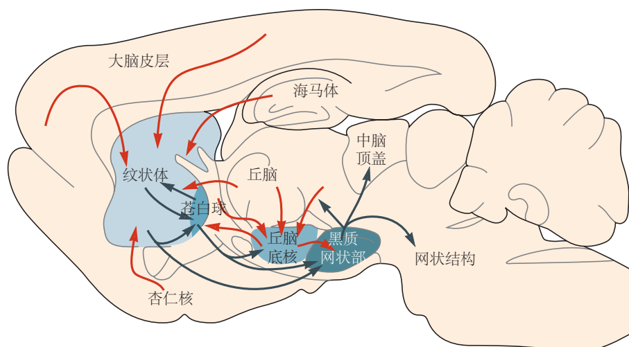
图 38.1.1: 哺乳动物基底神经网络的主要输入连接、内部连接和输出连接。主输入核是纹状体、丘脑底核和黑质致密部（未显示）。它们直接接收来自大脑皮层、边缘结构（杏仁核和海马体）、丘脑的输入。主输出核是黑质网状部和内侧苍白球/脚内核（未显示）。外侧苍白球被归类为内部核，因为它的大部分连接都与其他基底核相连。结构显示在啮齿类动物大脑的矢状图上。红色和深灰色箭头分别表示兴奋性连接和抑制性连接。
